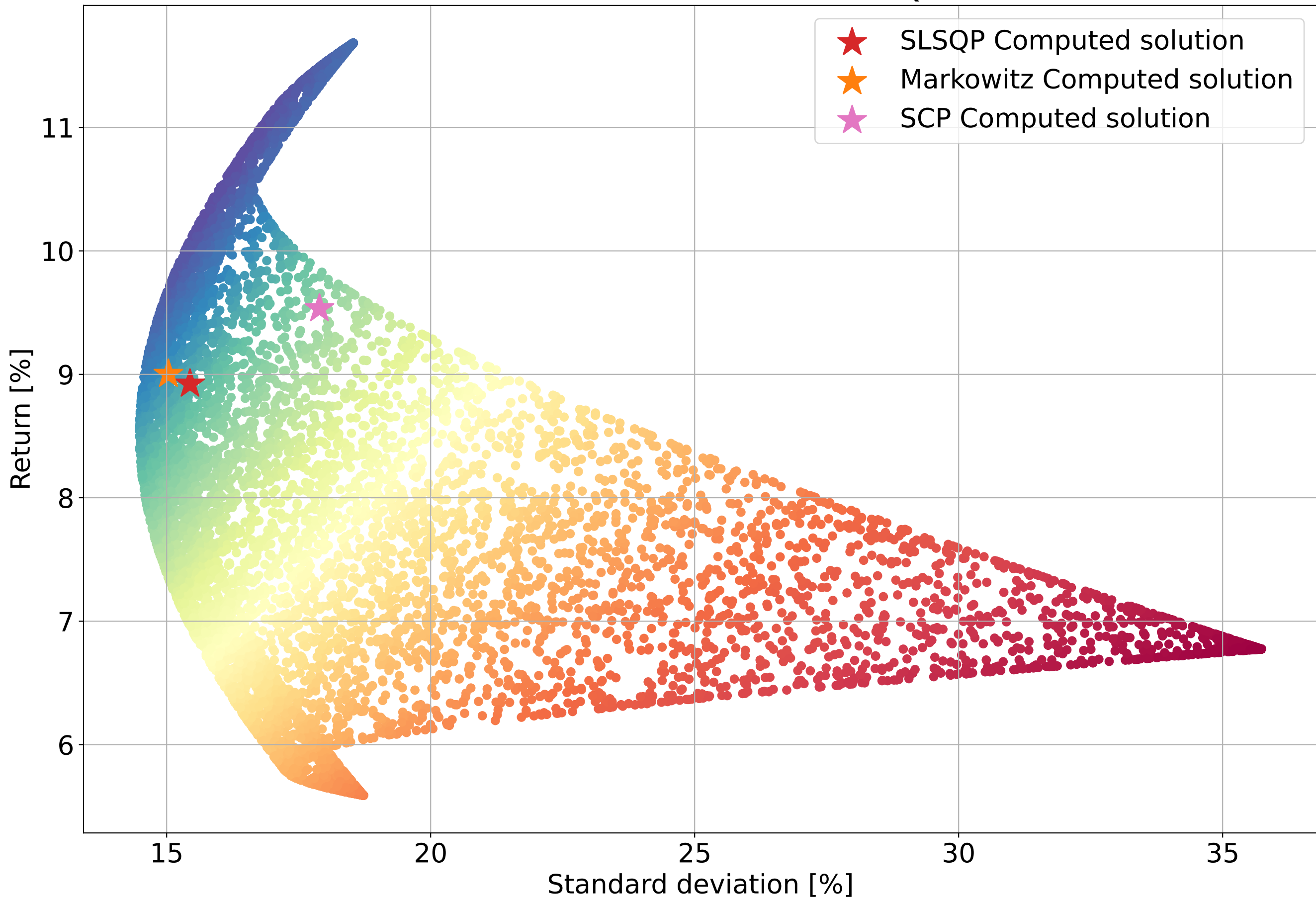
Efficient Frontier: Markowitz vs SLSQP vs SCP
