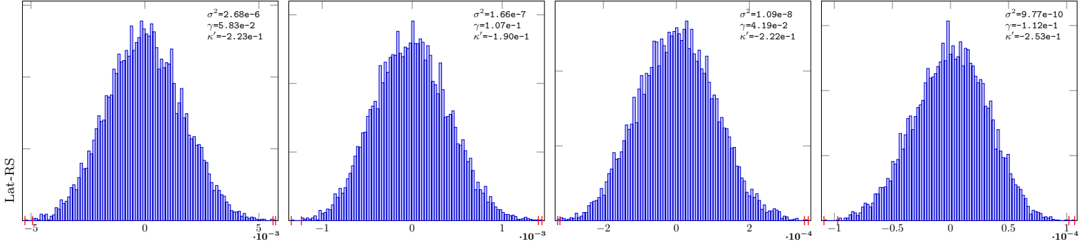
Gaussian-2-Lat-RSB-10
