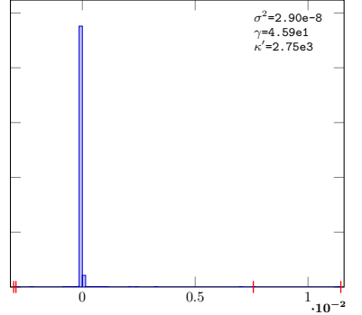
Gaussian-2-Lat-RpvRSB-16
