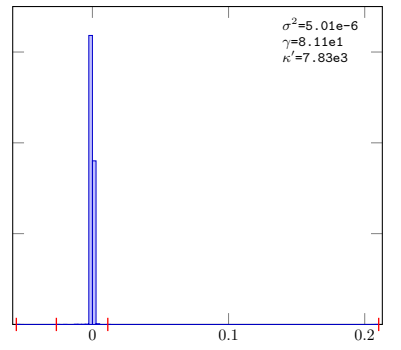
Gaussian-2-Lat-RpvRSB-16
