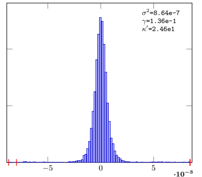
PieceLinGauss-32-Lat-RpvRSB-16
