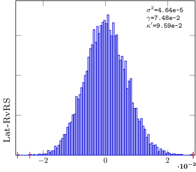
PieceLinGauss-32-Lat-RvRSB-10
