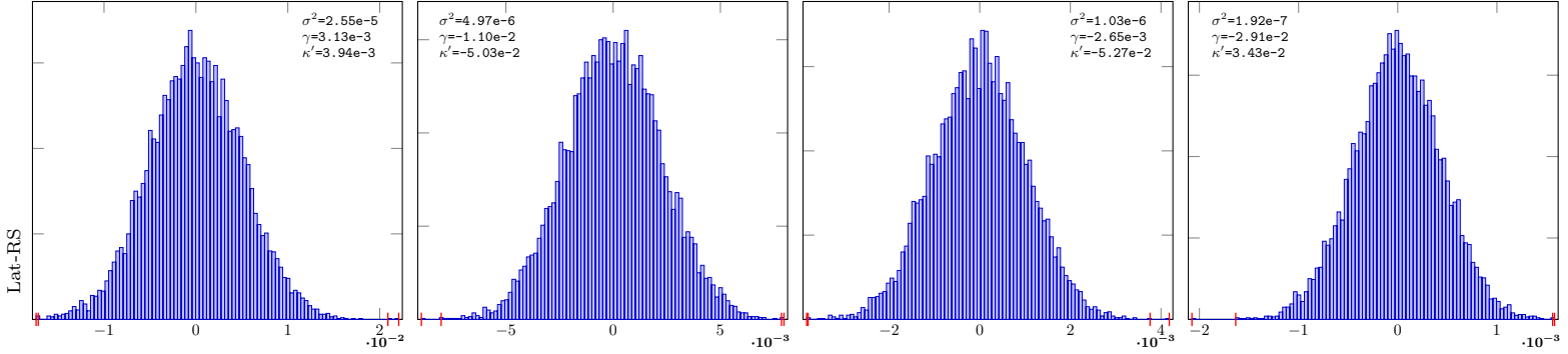
PieceLinGauss-32-Lat-RSB-10
