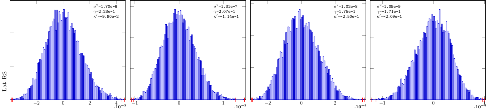
PieceLinGauss-2-Lat-RSB-10
