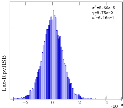
PieceLinGauss-32-Lat-RpvRSB-10
