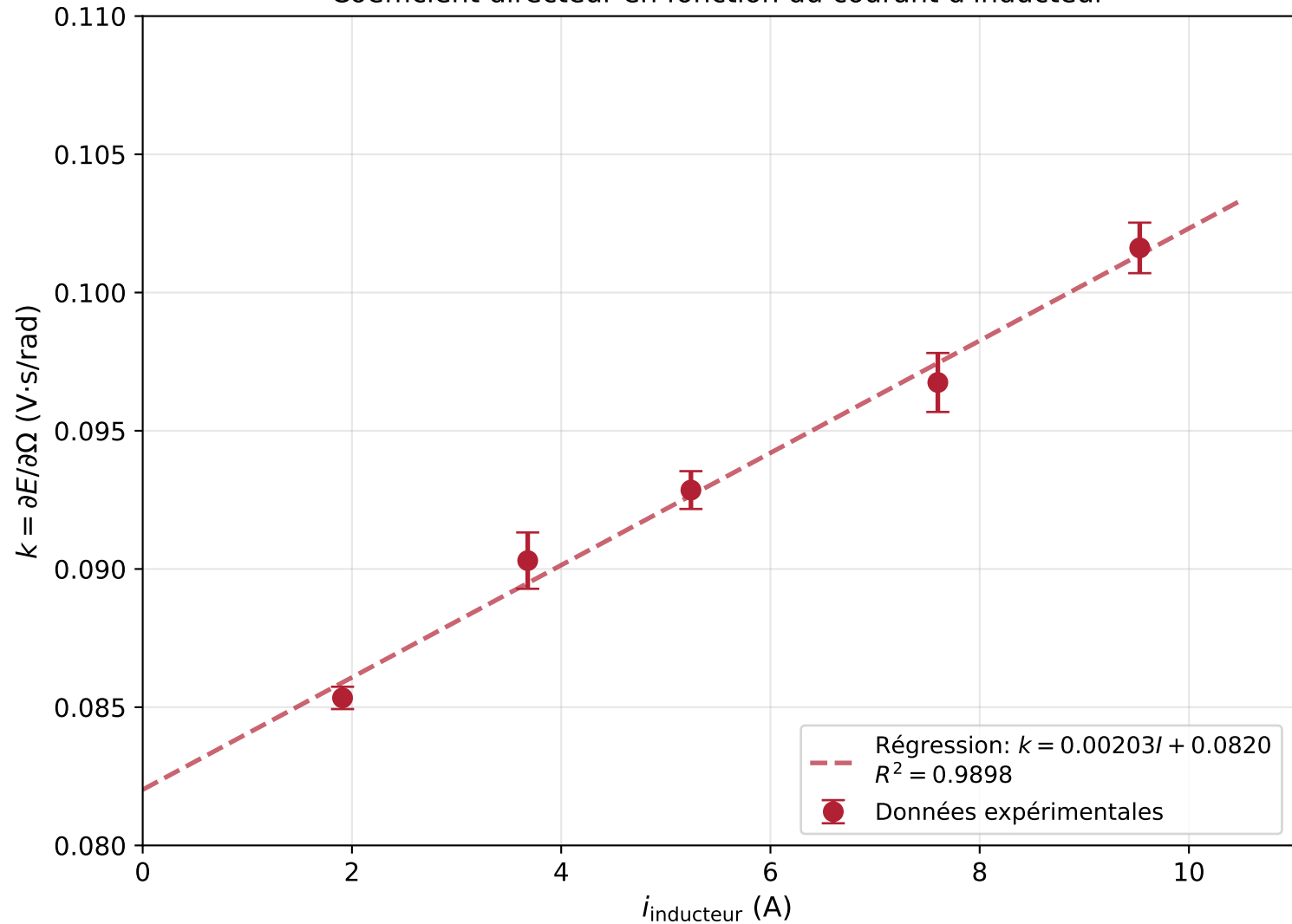
Coefficient directeur en fonction du courant d'inducteur
