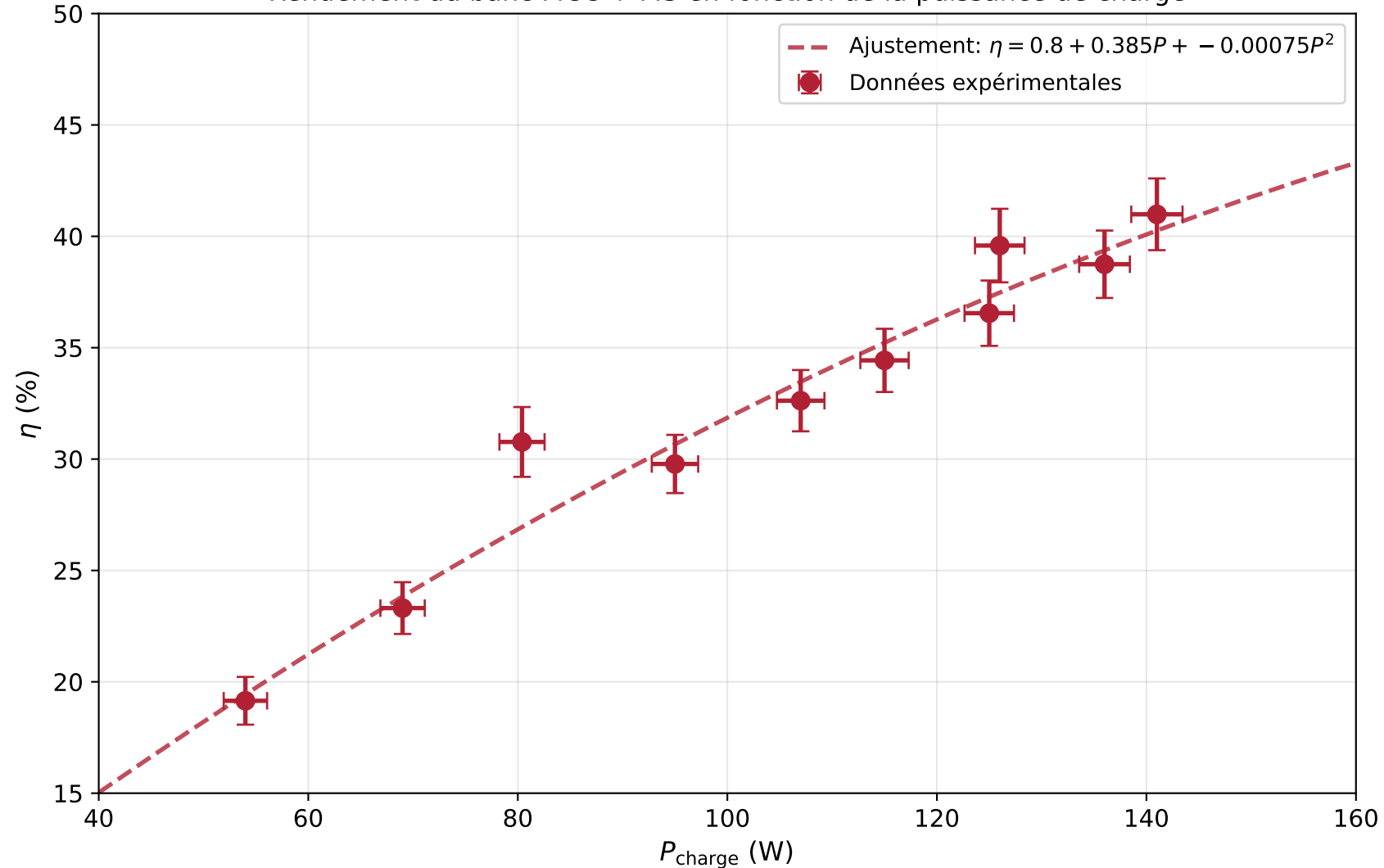
Rendement du banc MCC + MS en fonction de la puissance de charge
