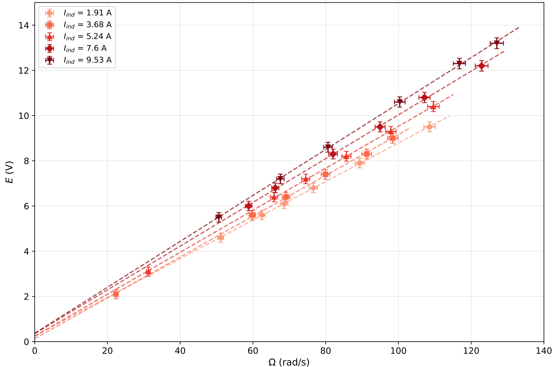
Force électromotrice induite en fonction de la vitesse de rotation
