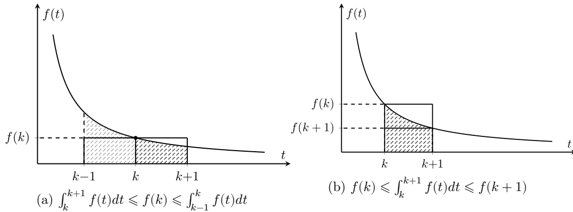
FIGURE 2.2 : Les deux versions de l'encadrement fondamental utilisé dans les comparaison séries-intégrales.
