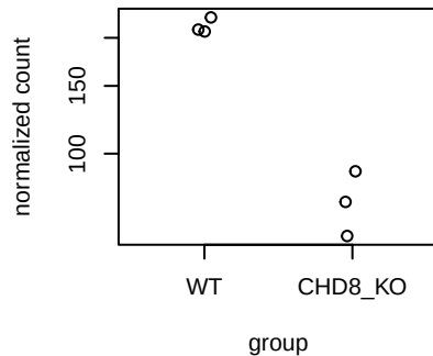
ENSMUSG000002076161
