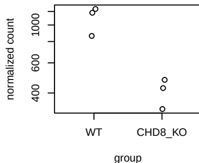
ENSMUSG00000036216
