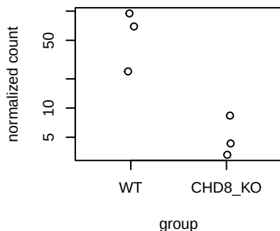
ENSMUSG00000117294
