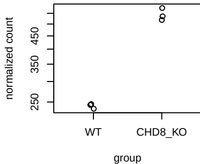
ENSMUSG00000033792
