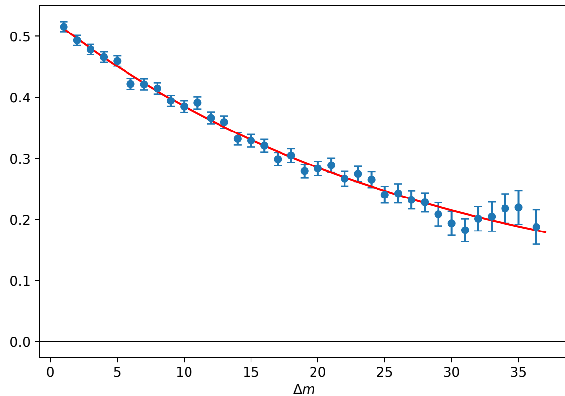
(d) \alpha = 0,97
