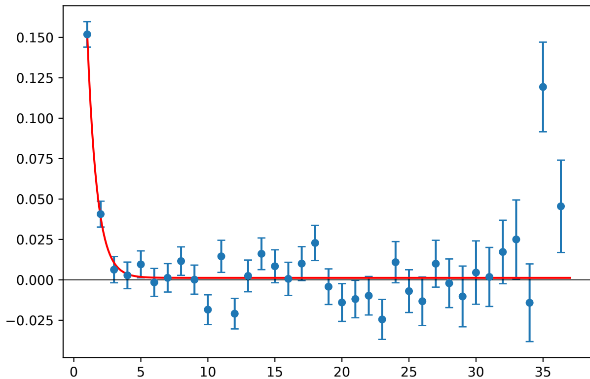
(c) \alpha = 0,87
