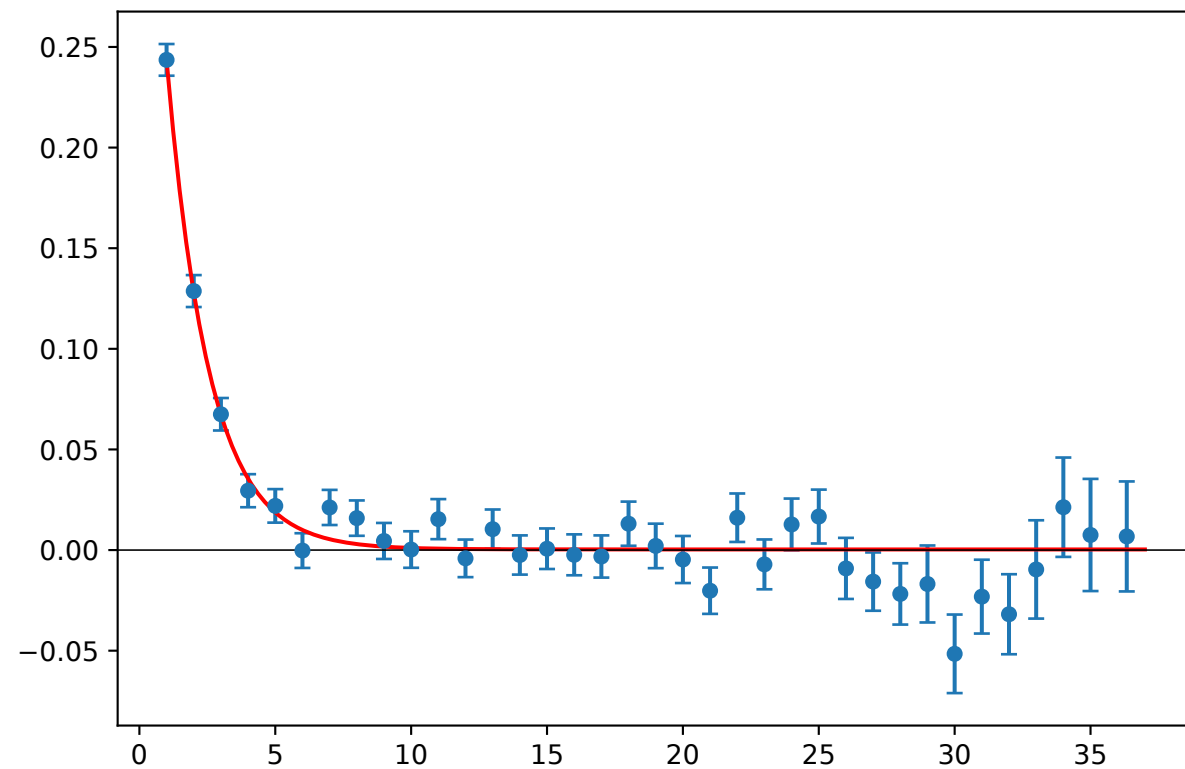
(d) \alpha = 0,97
