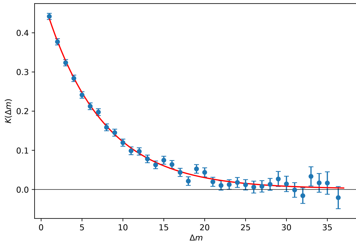
(c) \alpha = 0,87
