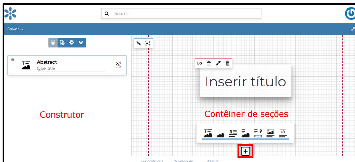
Figura 2. Interface gráfica de criação do Geostory em destaque o botão de mais que adiciona seções à página.
