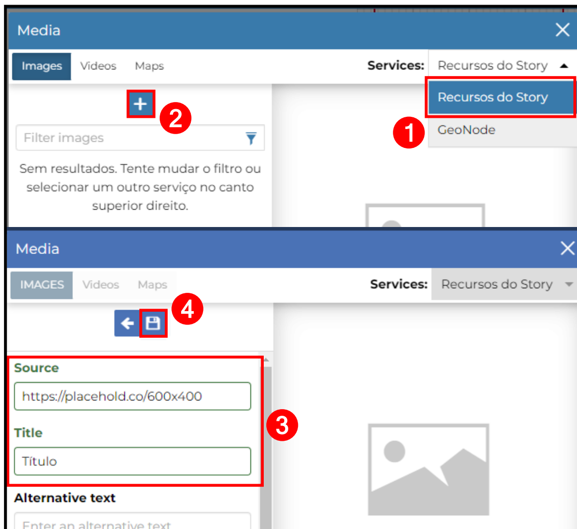
Figura 5. Interface gráfica de inserção de mídias externas.
