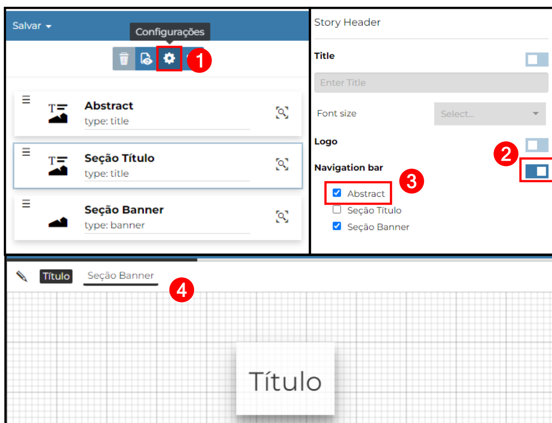
Figura 8. Configuração da barra de navegação de um Geostory.
