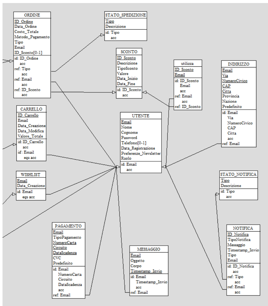
Figura 3.4: Schema Logico 2/2.
