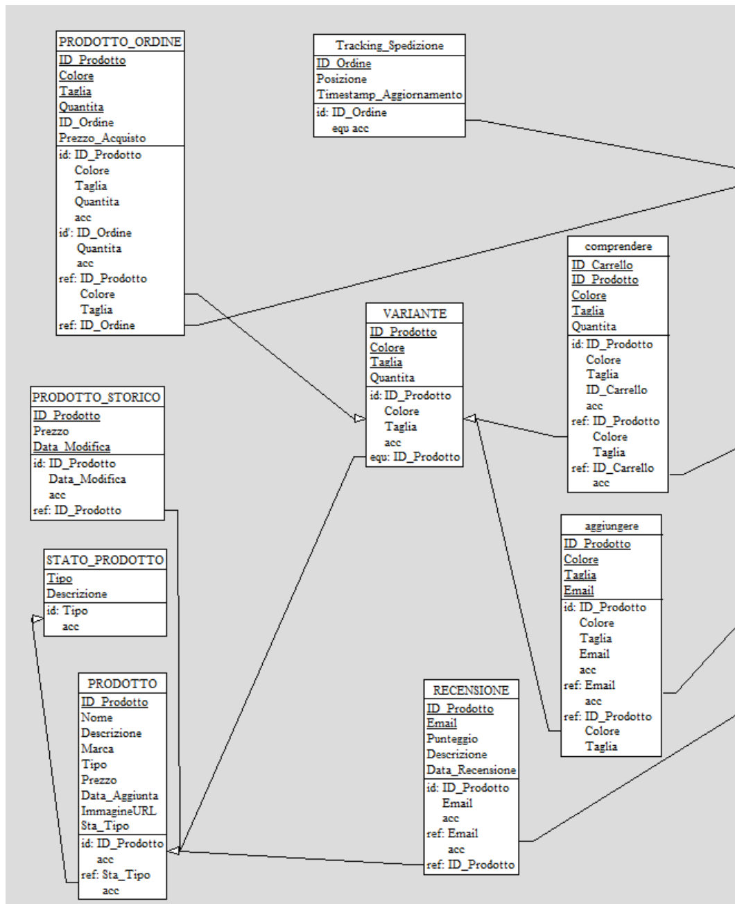
Figura 3.3: Schema Logico 1/2.
