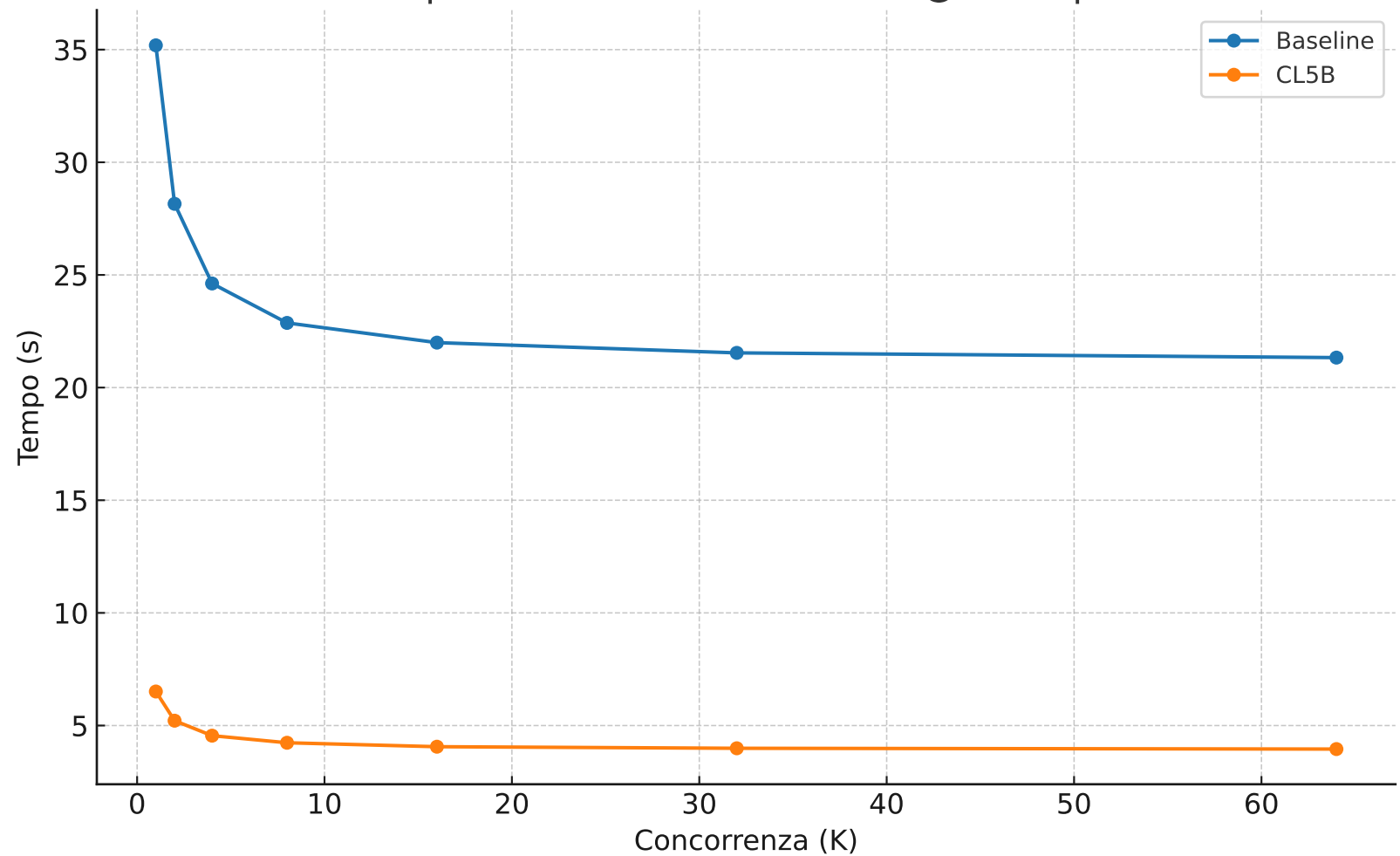
Cap 128.00 KB — RTT 35 ms @20 Mbps
