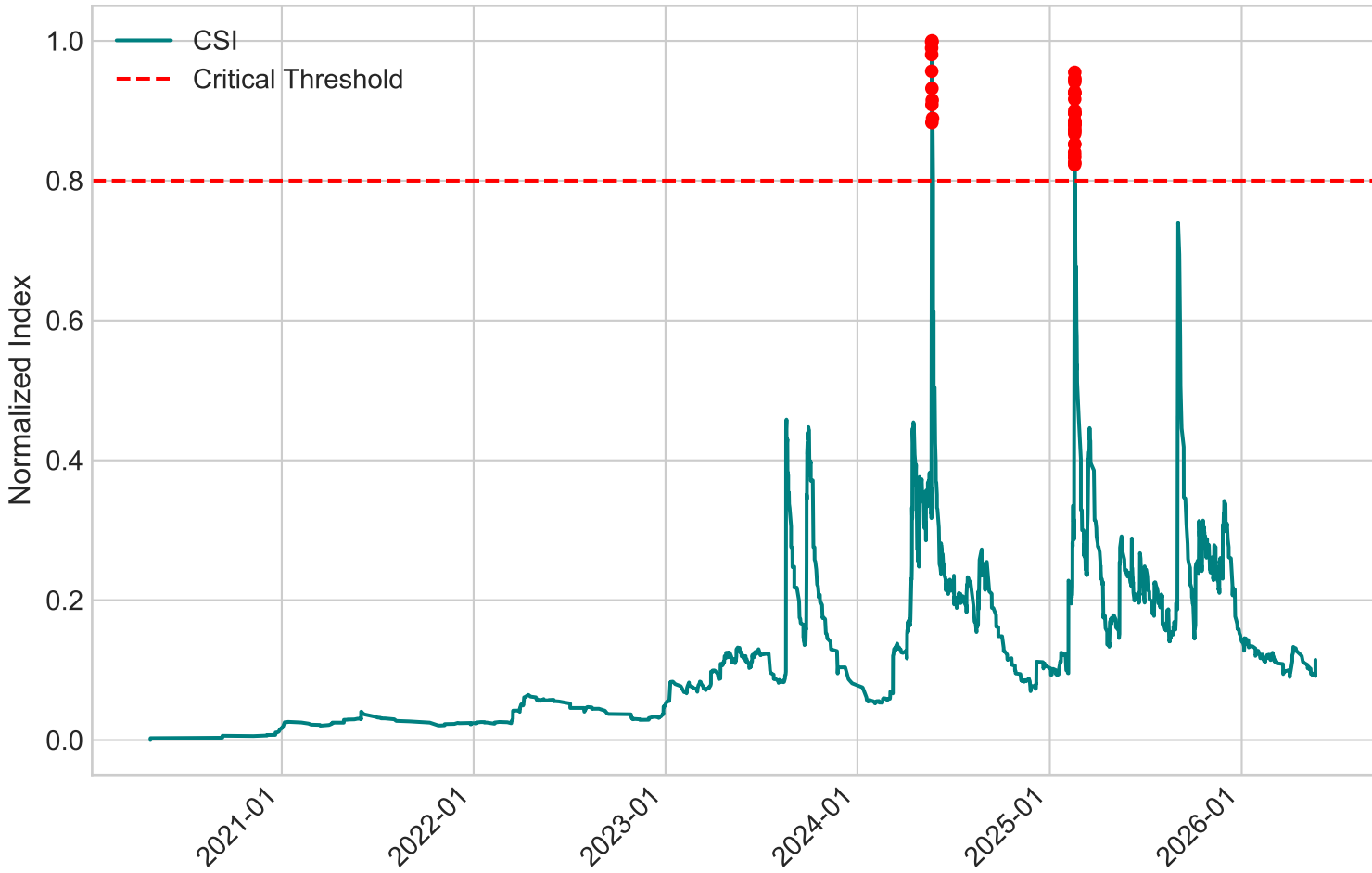
(D) Critical Seismicity Index (CSI)
