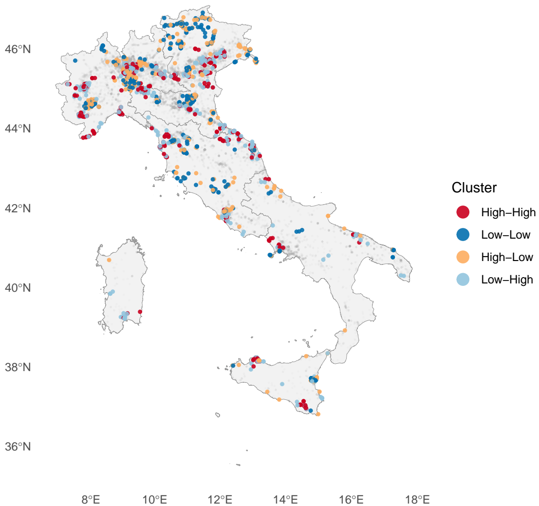
Mappa Aggregata: Cluster LISA Locali (W_strict)
