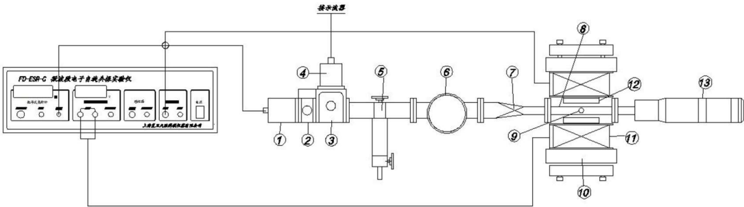
图 11 FD-ESR-C 型微波段电子自旋共振实验仪结构示意图
