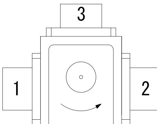
图 7 环行器结构
