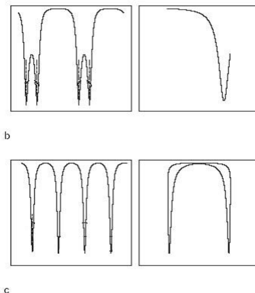
图 11 示波器观察电子自旋共振信号
