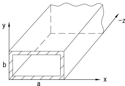
图 3 矩形波导管
