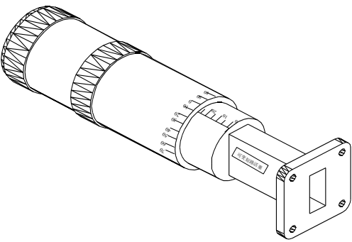
图10 短路活塞装置图
