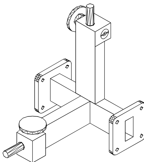
图 9 双 T 接头调配器
