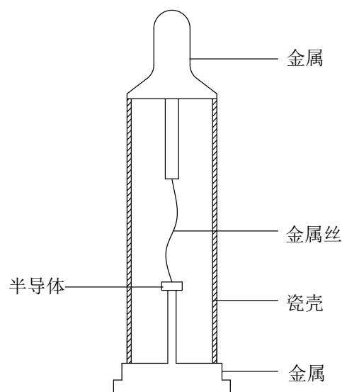
图 8 晶体检波器结构
