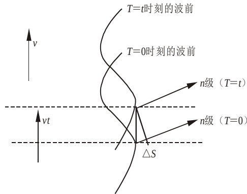
图 2 衍射光线在 y 方向上的位移量
