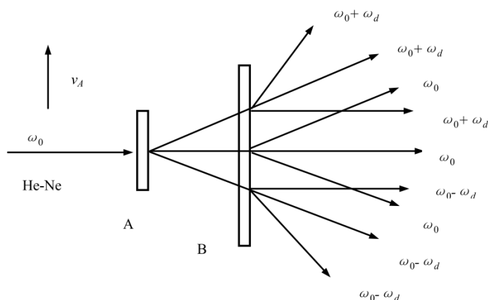
图 4 激光通过双光栅后所形成的衍射光
