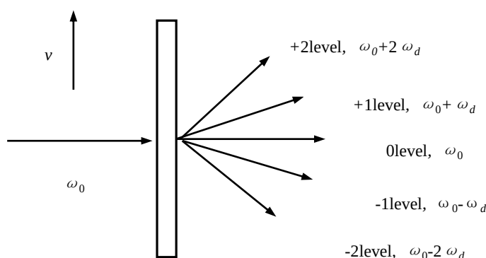
图 3 移动光栅的多普勒频移
