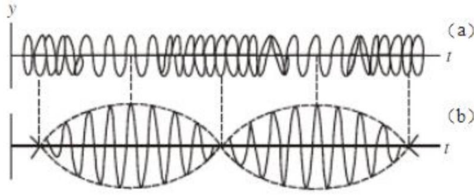
图 5 频差较小的两列光波叠加形成“拍”
