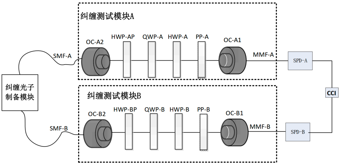
图 2: 测试模块的完整光路系统（来自讲义）
