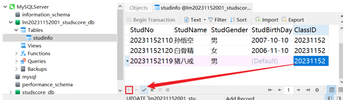
图 1- 6 添加记录
