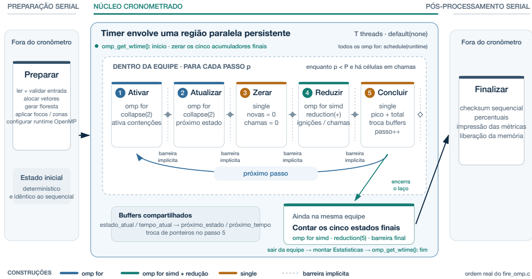
Figura 1: Fluxo exato da versão OpenMP. O cronômetro começa antes da região paralela persistente, inclui todas as fases dos passos e a contagem final, e termina após a consolidação das estatísticas. Os separadores pontilhados representam barreiras implícitas.
