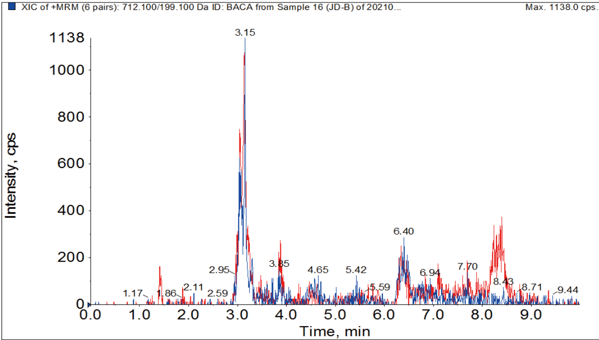
图1 空白鸡蛋 (杆菌肽A) 特征离子质量色谱图
