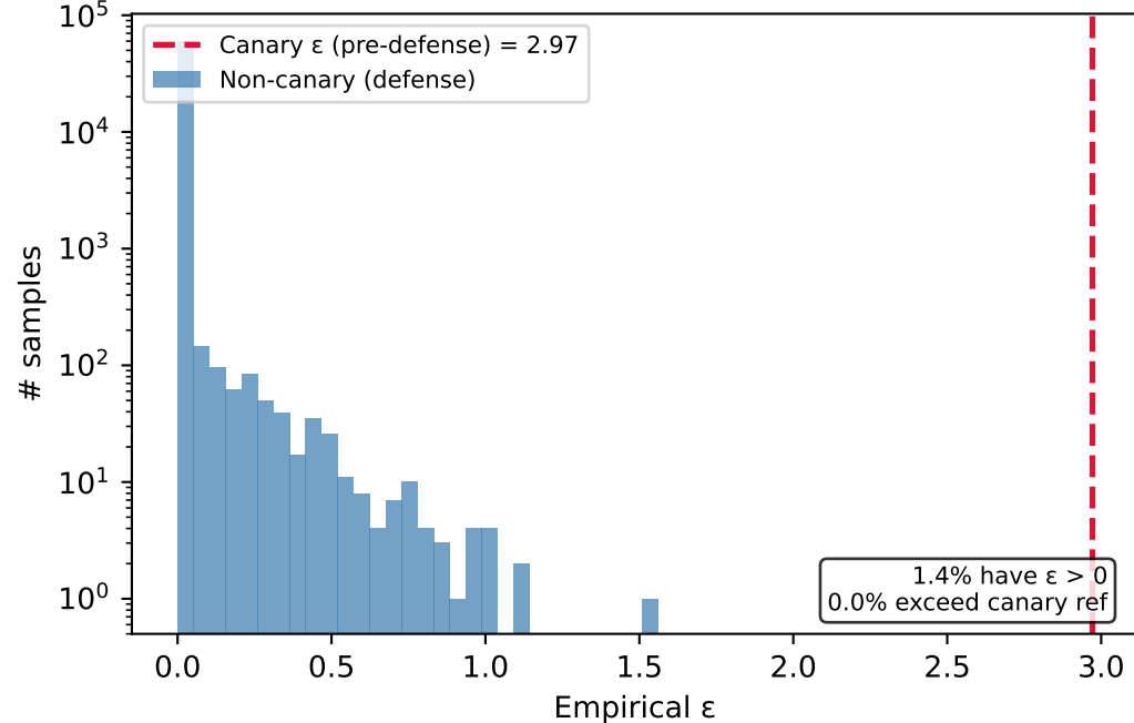
CP 50% holdout (valid lb)
