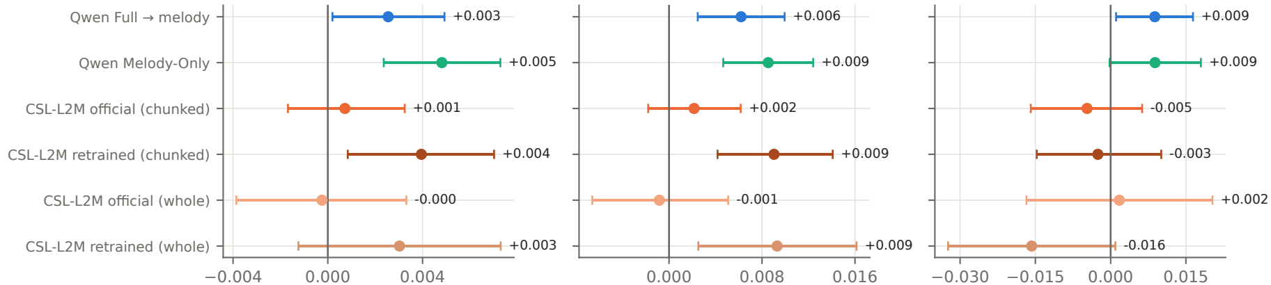
melody (1-LCS)
