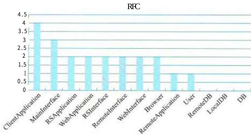
图10-23 Web读写系统各模块 R F C 度量结果
