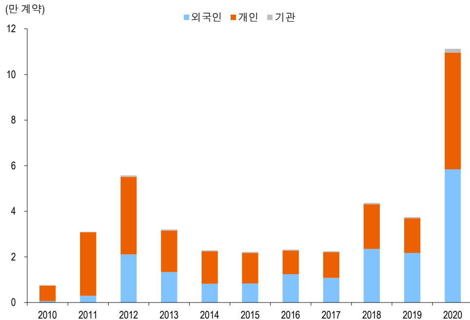
연도별 CME 연계 KOSPI200 야간선물 주체 간 일 평균 거래량(~2020년 3월)
