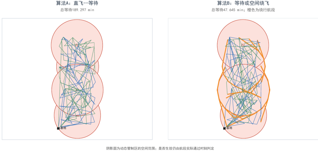
图 5 Case 2 中算法 A 与算法 B 的规划航迹对比（橙色折线表示算法 B 的绕飞航段）
