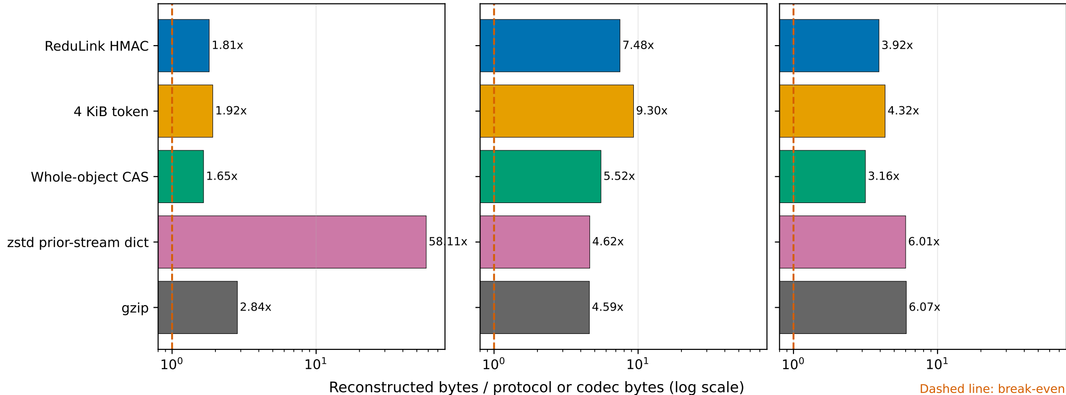
Nginx
