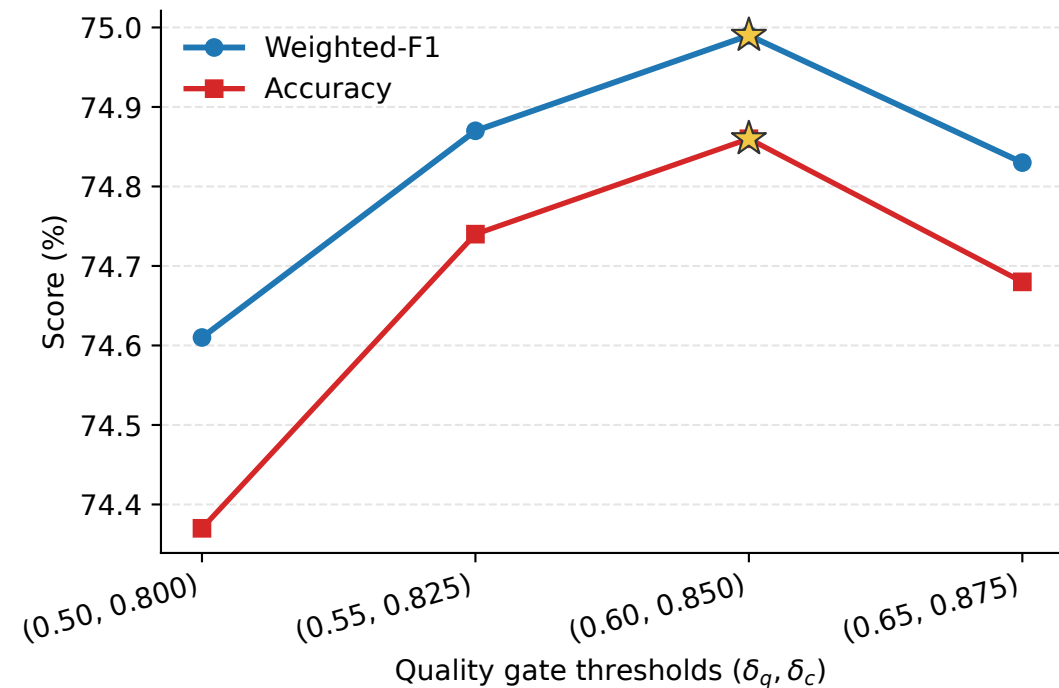
IEMOCAP
