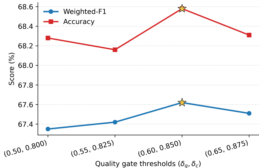
MELD
