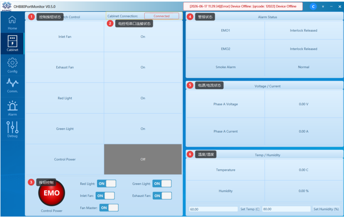
图 4-17 Cabinet 界面整体布局与编号标注（正文中的【1】至【6】均对应本图编号）
