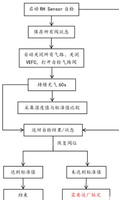
图 4-22 SH85 周期自检固件流程图
