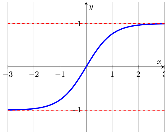
Graphes de \tanh(x)
