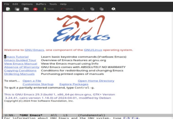
Рисунок 1: Запуск Emacs
