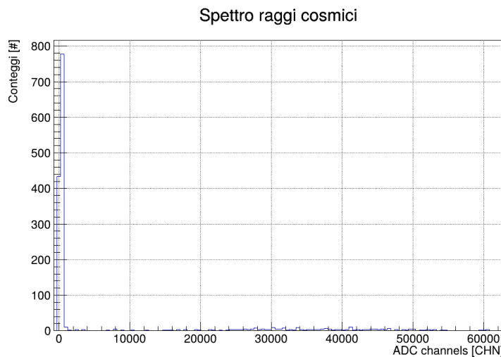
Fig. 3.1: Istogramma di conteggi per numero di canale per i muoni cosmici completo ( G_{ampl} = 28\text{dB} e V_{bias} = 54V ).
