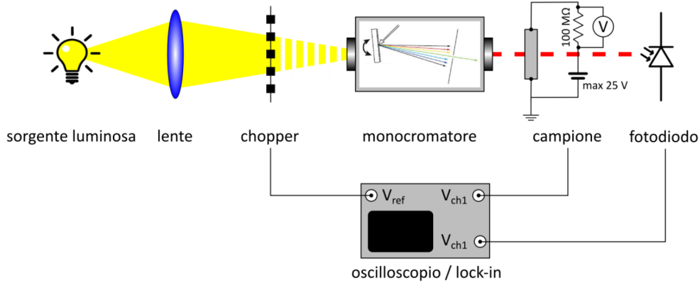
Fig. 1.1: Schema dell'apparato sperimentale.
