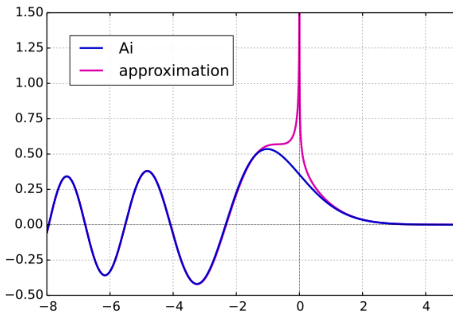
Fig. 14.2: Grafico di \text{Re}(Ai(z)) (in blu) e dei due andamenti asintotici (in rosa)
