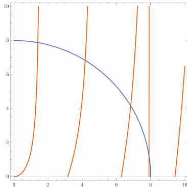
Fig. 3.1: Soluzioni per le autofunzioni pari
