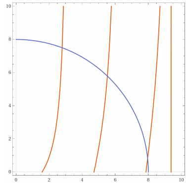
Fig. 3.2: Soluzioni per le autofunzioni dispari
