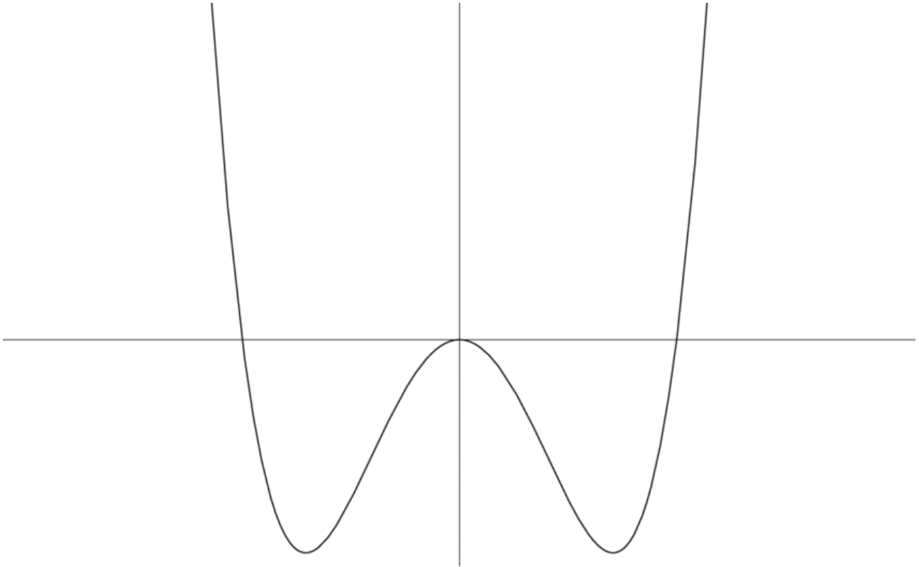
Fig. 3.3: Potenziale V(x) = x^4 - x^2 , un esempio di potenziale a sombrero
