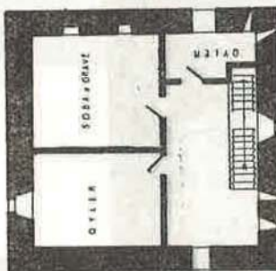
PLANIMETRIA E KATIT QUTE
