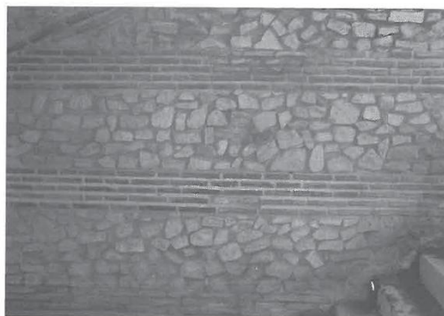
Fig. 16. Muraturë e përzjerë me pesë radhë tullash
