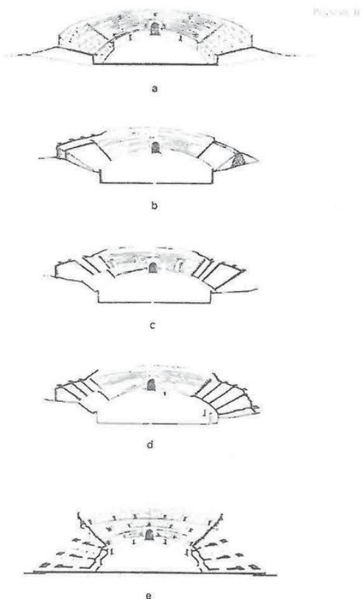
Fig. 1. Tipologjia e amfiteatrove (sipas Golvin)
