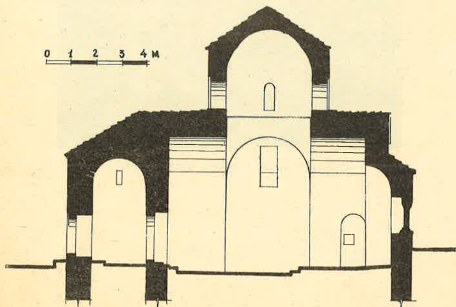
Fig. 2 - Prerje gjatësore
