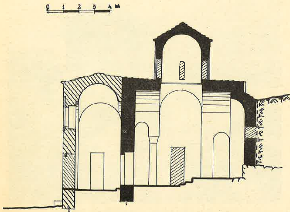
Fig. 17 - Prerja gjatësore
