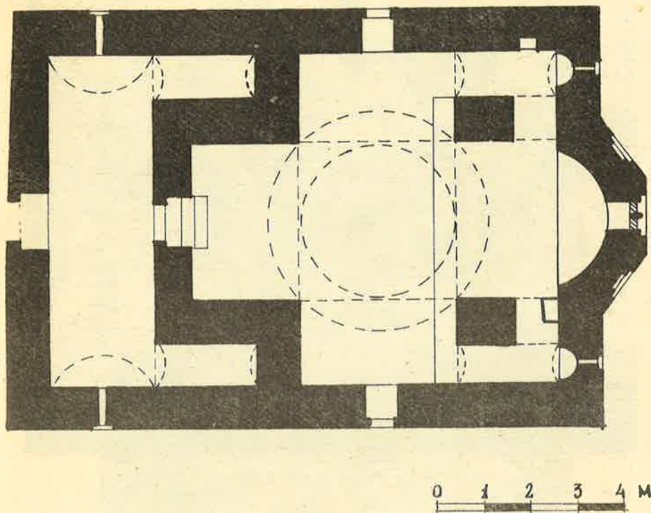
Fig. 1. - Planimetria e kishës së Kosinës
