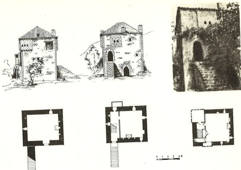
Fig. 11. Kullë me dy hyrje, Kurdari, Mat.
