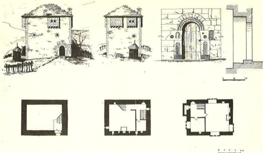
Fig. 1 - Kullë në fshatin Macukull ÷ Mat.
