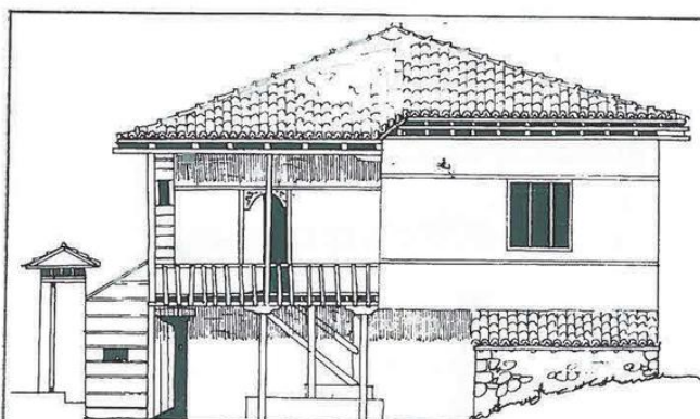
PAMJE KRYESORE (PARA RESTAURIMIT)
