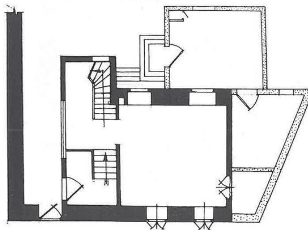
PLANIMETRIA E KATIT PERDHE
