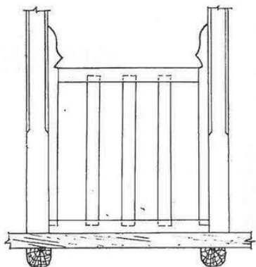
DETAJ I "PARMAKLEKUT"
