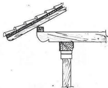
DETAJ I STREHES SE ÇARDAKUT
