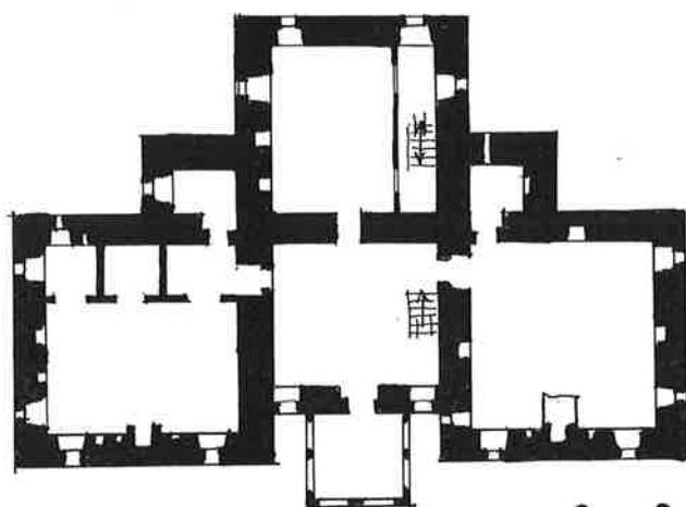
FIG. 1. — Popçisht-Korcë Habitation à kulle. T. — Tourelle
