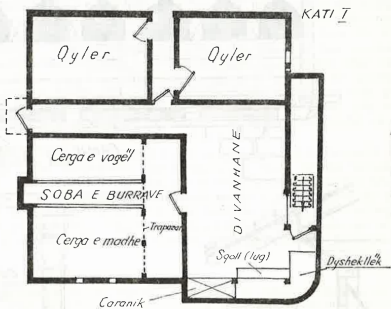
Çardak i vjetër — Lëbushë.
