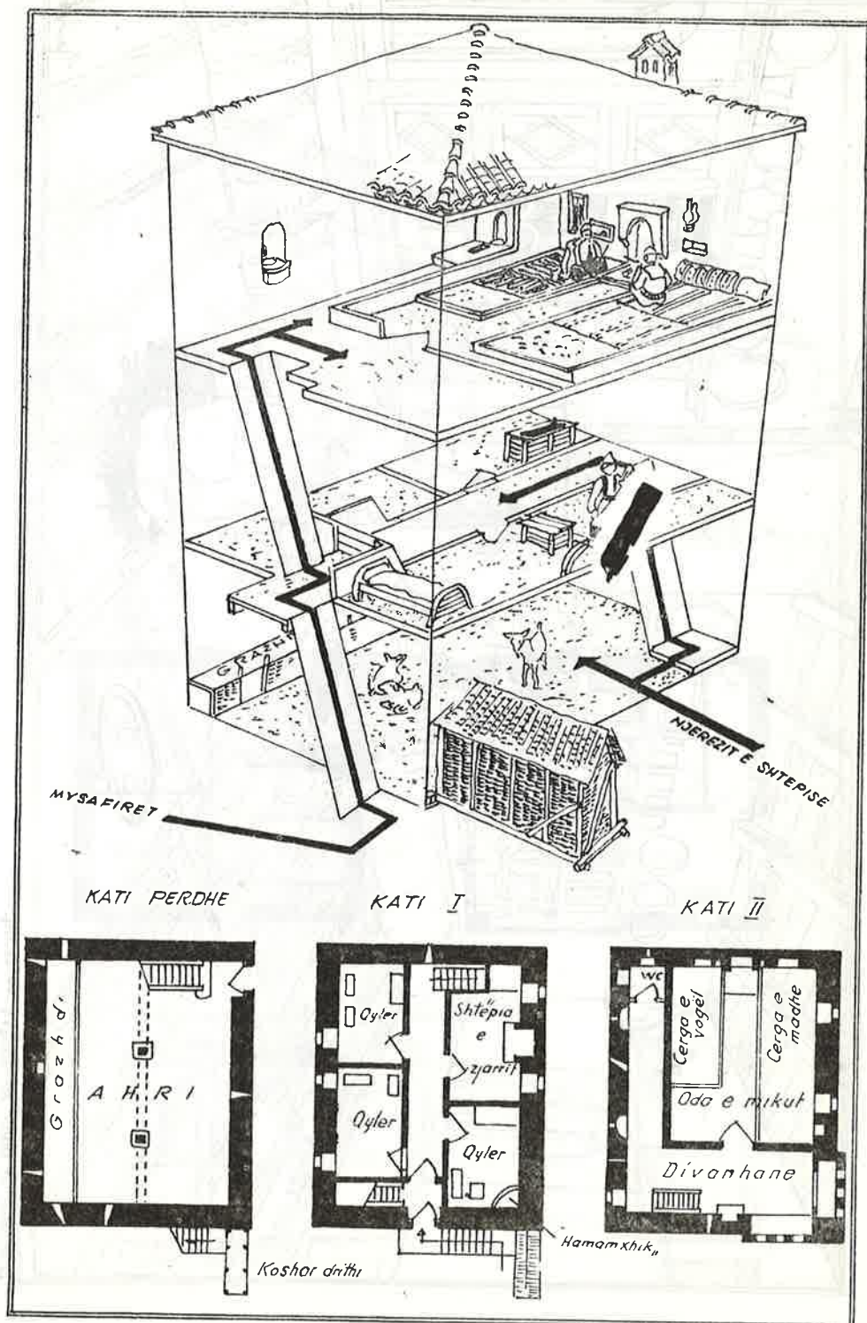
Skema funksionale dhe kompozicionale e kullës trikatëshe (Sipas M. Krasniqit).
