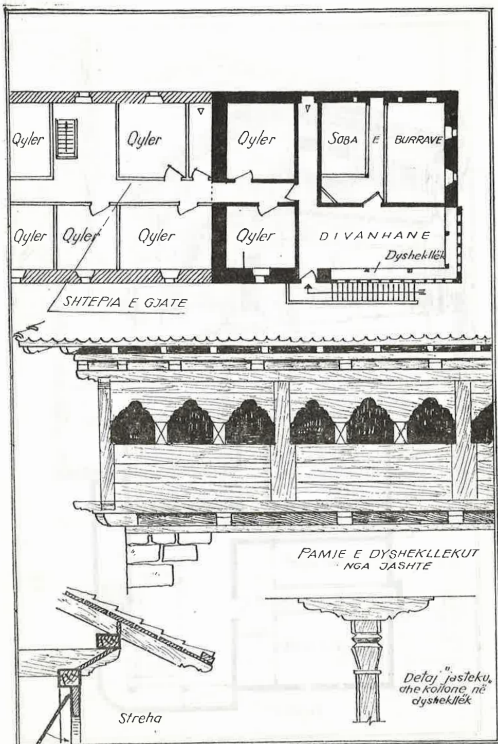
Banesë dykatëshe — Pobërgjë.
