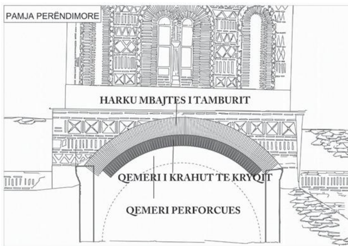
Fig. 17. Skema konstruktive e krahëve të kryqit
