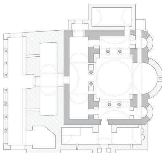
Fig. 2. Planimetria e kishës me fazat e ndryshme ndërtimore
