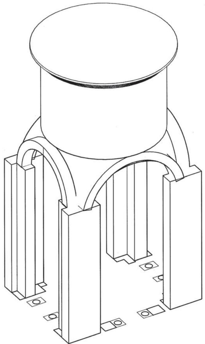
Fig. 16. Skema konstruktive e pjesës qendrore
