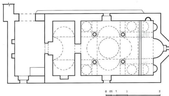
Fig. 19. Manastiri i Shën Qiriakut dhe Julitës, Dhuvjan, planimetria e kishës së manastirit
