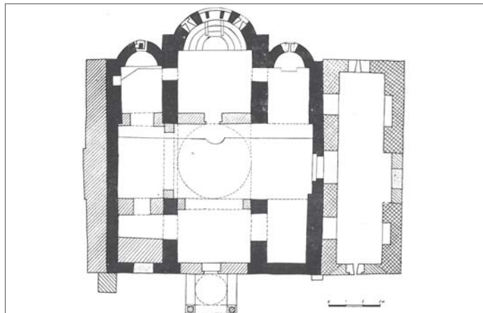
Fig. 3. Planimetria
