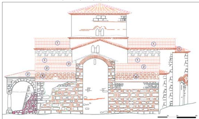
Fig. 39. Propozimi për pamjen jugore të kishës
