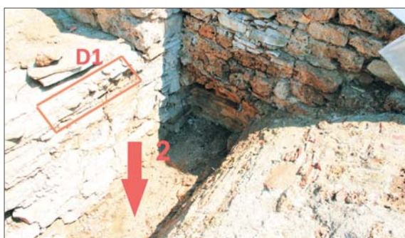
Fig. 20. Zbulimi i ullikut ndërmjet mbulesës së fazës së parë dhe shtesës jugore në anën perëndimore
