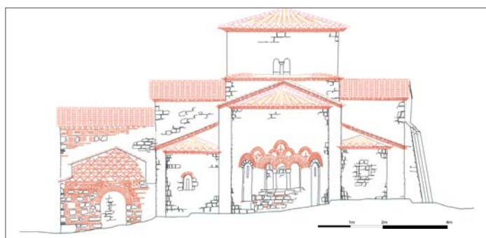
Fig. 38. Propozimi për pamjen lindore të kishës
