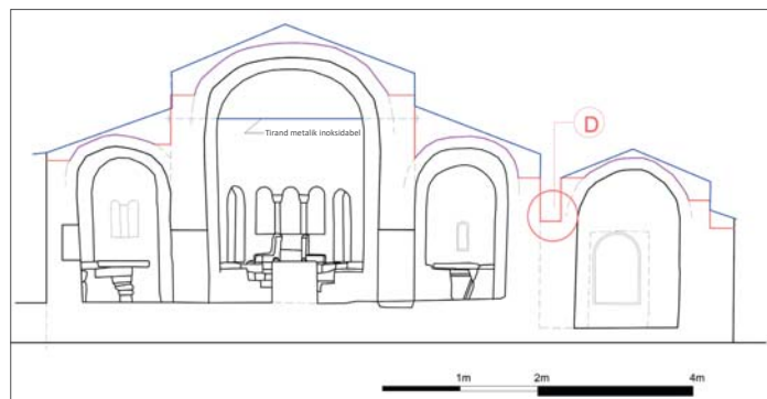
Fig. 28. Konfiguracioni i mbulesës fillestare të anës lindore
