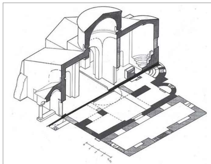
Fig. 4. Prerja aksometrike
