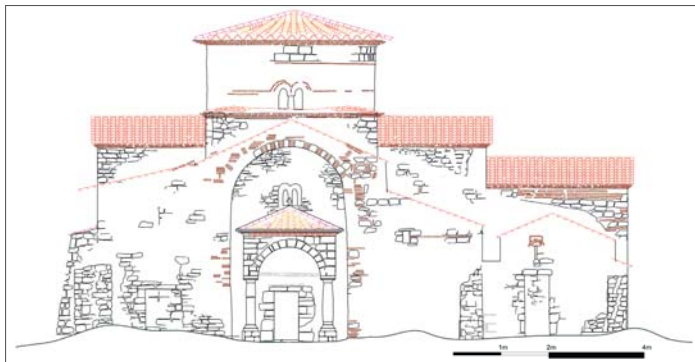
Fig. 37. Propozimi për pamjen perëndimore të kishës
