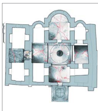
Fig. 14. Dëmtimet e sistemit të mbulesës
