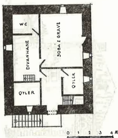
PLANIMETRIA E KATIT II
