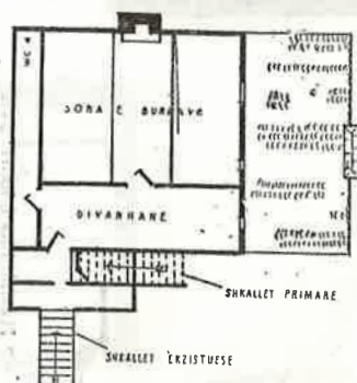
PLANIMETRIA E KATIT II-TE
