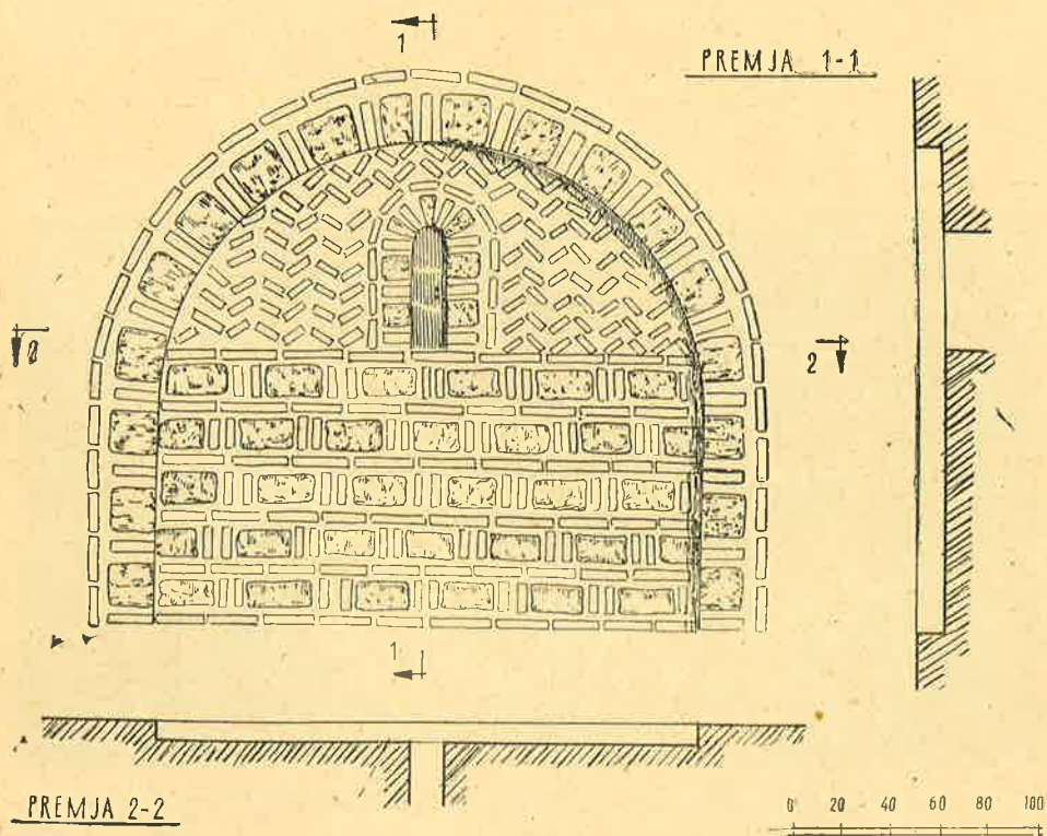
Fig. 11. Nikja në murin jugor
