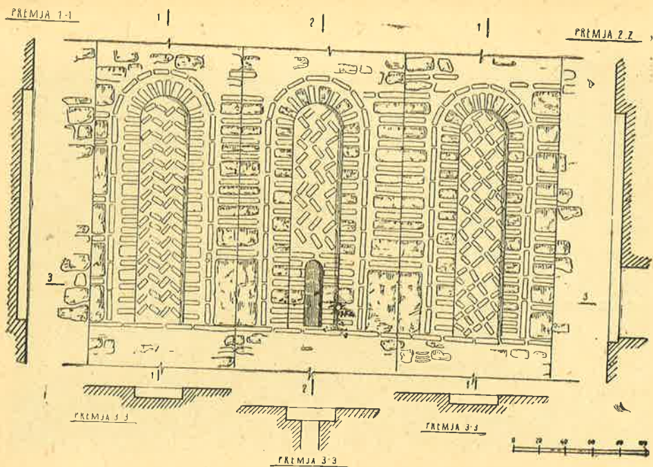
Fig. 10. Niket e faqeve të apsidës
