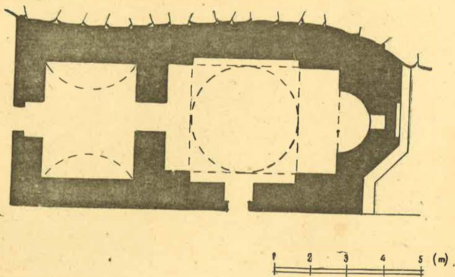
Fig. 4. Planimetria e kishës së Shën Mihillit në Berat
