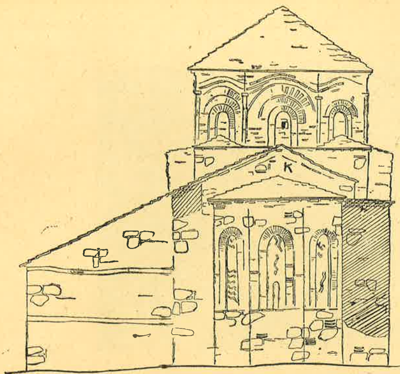
Fig. 5. Pamja lindore në gjendjen e sotme me shtesat dhe meremetimet e mëvonshme.
