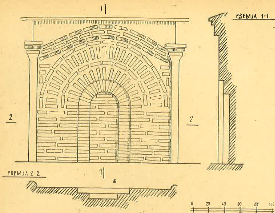
Fig. 12. Faqja e tamburit
