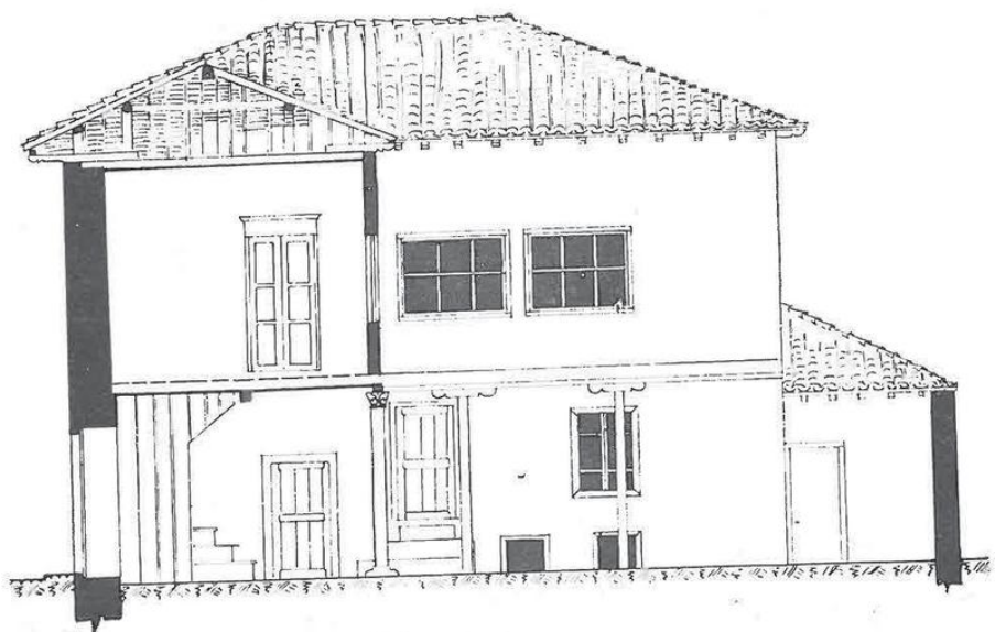
PRERJE B-B
