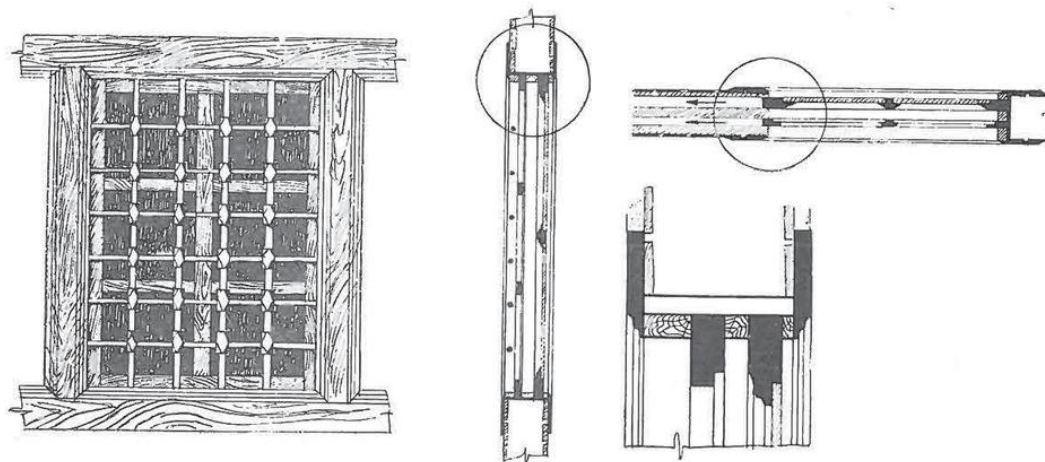
DETAJ DRITAREJE
