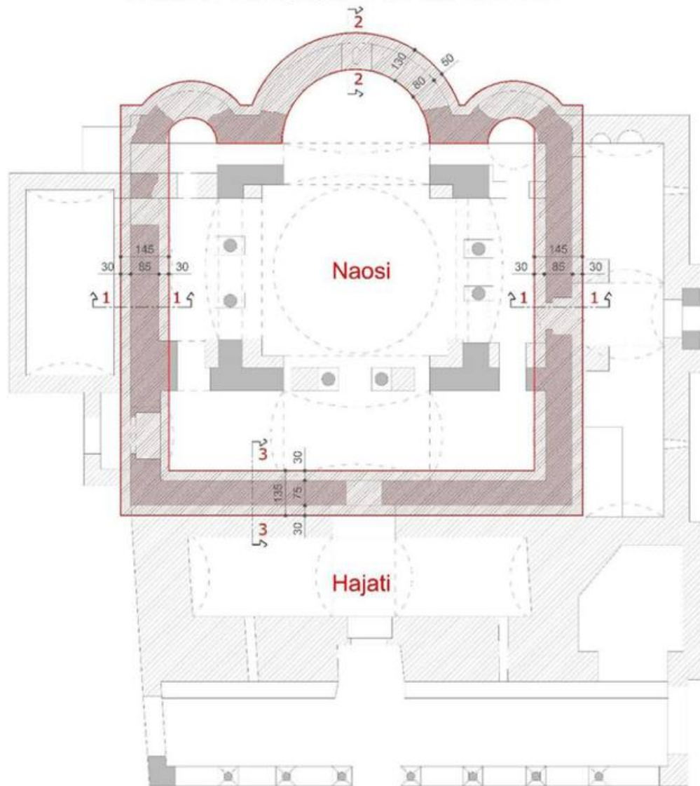
PLANI I PËRFORCIMIT TË THEMELEVE
