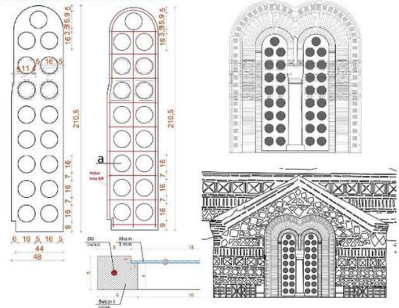
DIAFRAGMAT E FRONTONIEVE
