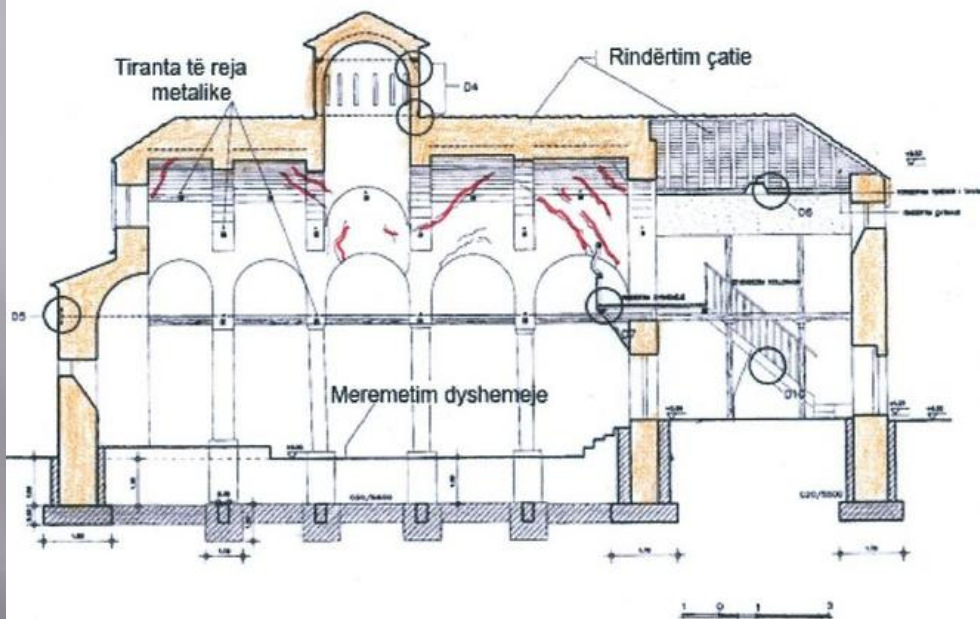
PRERJE GJATESORE
