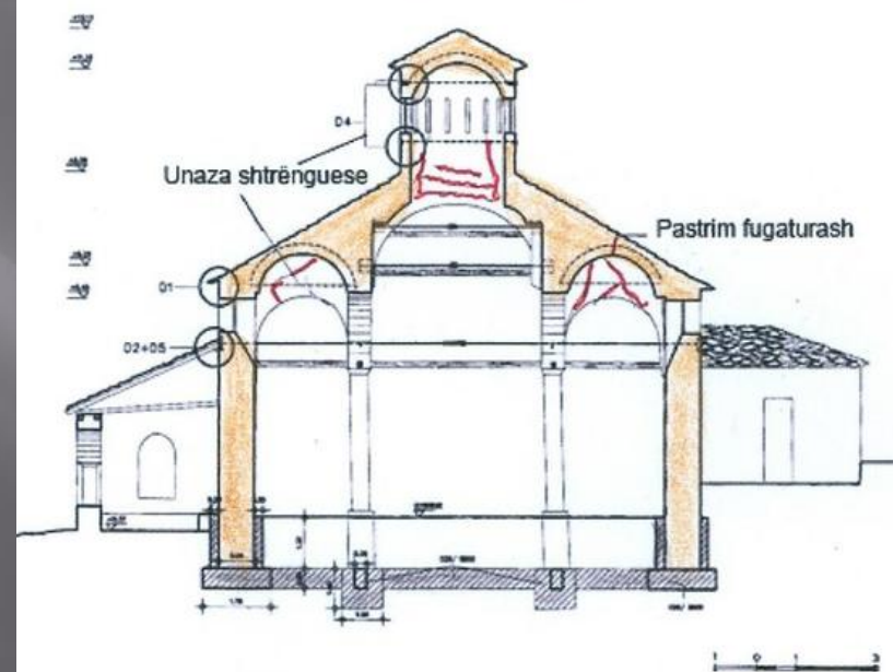
PRERJE TERTHORE
