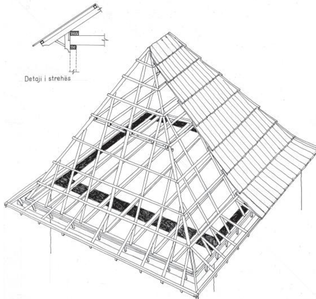
Fig. 60. Tamarë, Kelmend-Shkodër. Konstruksioni i një çatie të pjerrët. Mbulesa e lehtë me furde dërrase dhe pjerrësia e madhe për rrëshqitjen e borës i kanë dhënë mundësi ndërtuesve që të ngrejë një konstruksion të lehtë, pa harxhim të madh të lëndës drusore.
