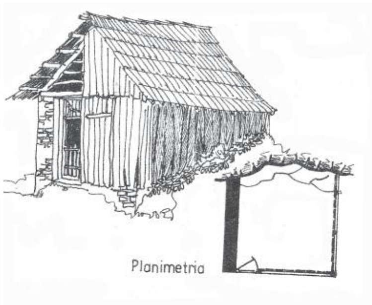
Fig. 297. Lenë, Martanesh-Mat. Kasolle gjaje.
