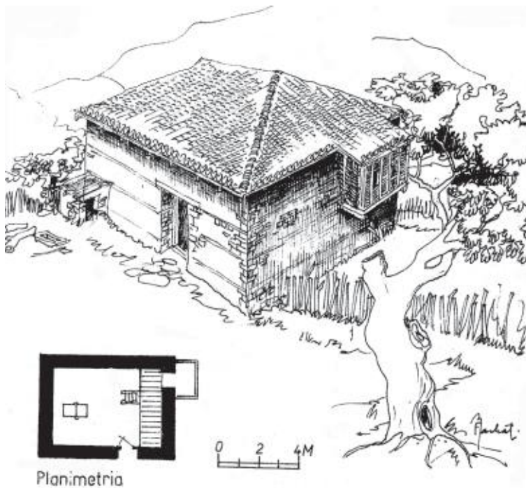
Fig. 362. Linzë, Ranzë-Tiranë. Banesë e thjeshtë njëkthinëshe përdhese e përdorur si shtëpi zjarri. Brenda mjedisit është ndërtuar mafili, për rritjen e sipërfaqes së banuar, i pajisur me një qoshk të dalë.
