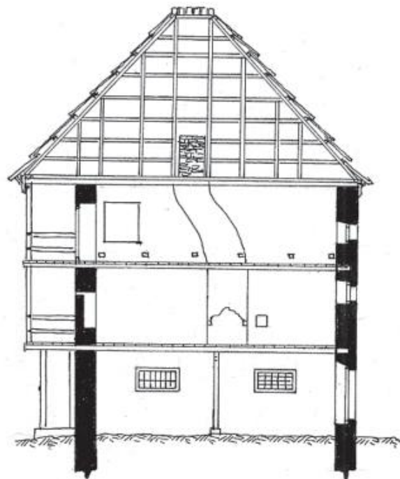
Prerje A-A
