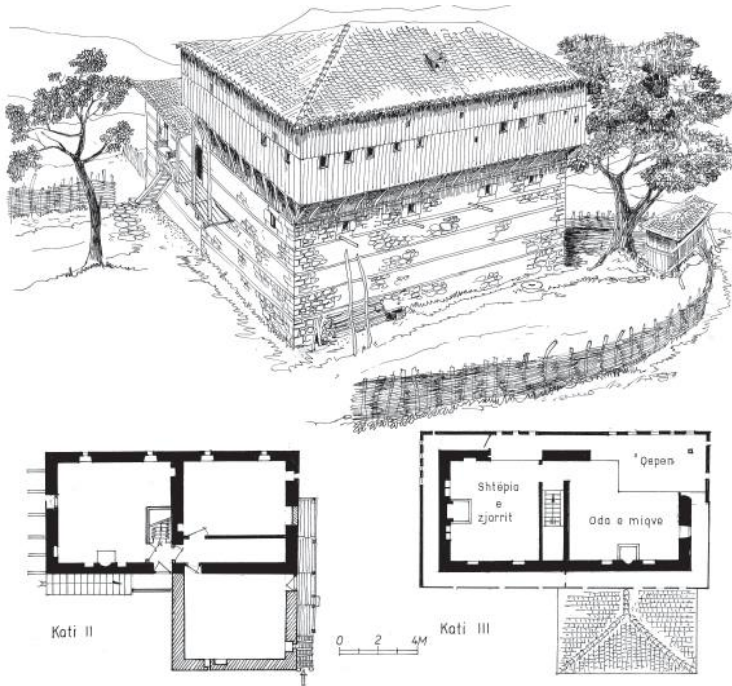
Fig. 436-437. Orenjë, Çermenikë-Librazhd. Skema dykthinëshe në kat ka gjetur një zgjidhje më organike, jo vetëm me shtimin e numrit të mjediseve por kryesisht me diferencimin funksional të tyre. Oda e miqve dallohet nga qepeni tepër i
