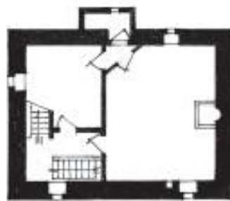
Kati II
