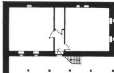
Kati përdhe
