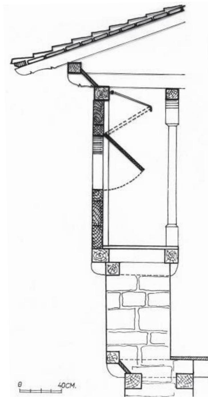
Fig. 173-174. Has-Kukës. Detaje konstruktive prej druri. Karakteristikë e konstruksioneve të tilla është vënia në dukje e strukturës mbajtëse. Çdo element i dukshëm i kësaj strukture, si bishtat e strehës, daljet e trarëve të tavanit ose të dyshemesë, jastëkët e kolonave etj, i nënshtrohen një përpunimi të lehtë por me vlera dekorative.
