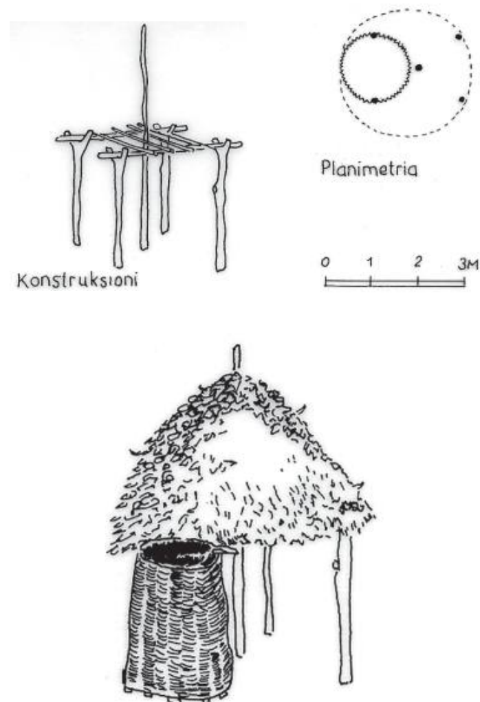
Fig. 32-33. Formë e thjeshtë e koshit të misrit, me planimetri rrethore dhe janë ndërtuar me gardh. Mbi të ngrihet mullari që mbron koshin dhe njëkohësisht krijon një strehë qëndrimi e pune.
