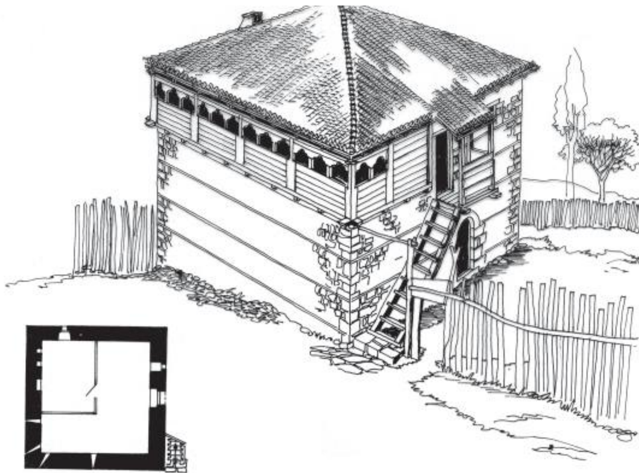
Kati përdhe
