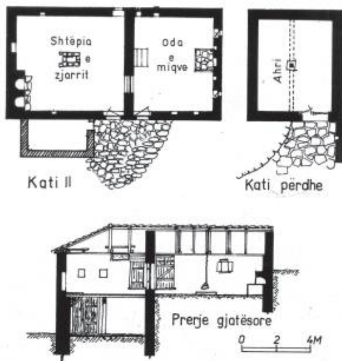
Fig. 74-75. Patalej, Malësia e Lezhës-Lezhë. Kompozimi vëllimor me gjysmëkat ka gjetur një përdorim të gjerë në banesat e ndërtuara në terrene të pjerrëta. Banesa e paraqitur është një shëmbull tipik. Secili mjedis ka hyrje të veçantë nga jashtë, por ndërlidhen edhe së brendëshmi ndërmjet tyre.
