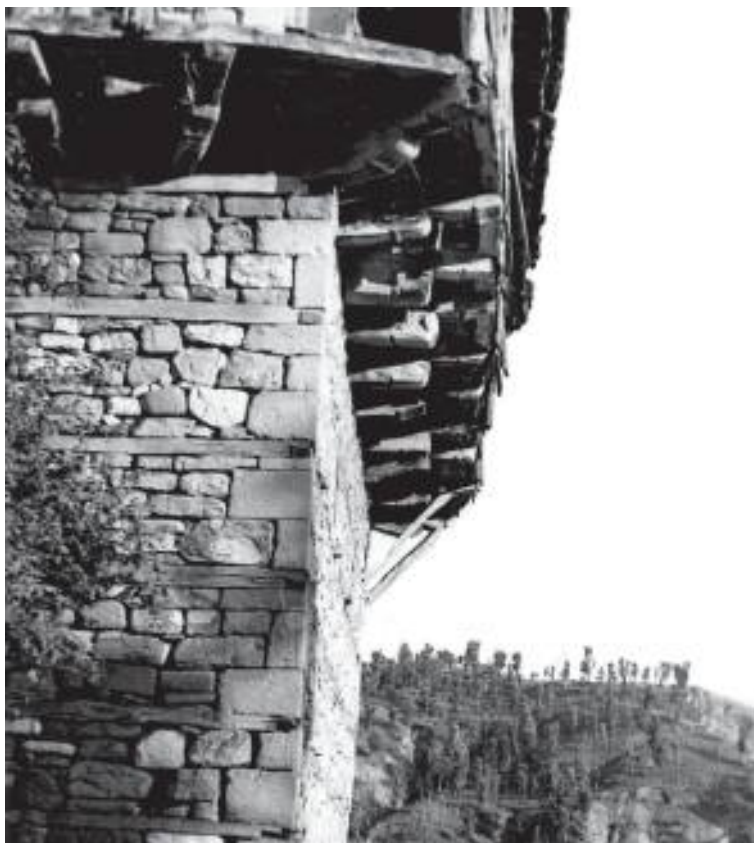
Fig. 493. Gur i Bardhë-Mat. Dalje konsol e muraturës së katit.
