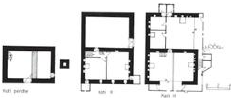
Fig. 431. Bastar i Mesëm, Malësia e Tiranës-Tiranë. I njëjti kriter i zhvillimit tërthor me rënien e terrenit të banesës, ka marrë trajtime të ndryshme të mjediseve të banuara. Galeria e mbyllur, telizi që e qarkon katin në dy anë, përmban qepenin e dhomës së miqe dhe atë të shtëpisë së zjarrit, të cilat kanë rritur në mënyrë të ndjeshme hapësirën e këtyre mjediseve. Në një fazë më të vonë, në shtëpinë e zjarrit, janë veçuar dy kthina fjetjeje dhe dhoma e miqe është ndarë në dy pjesë.
