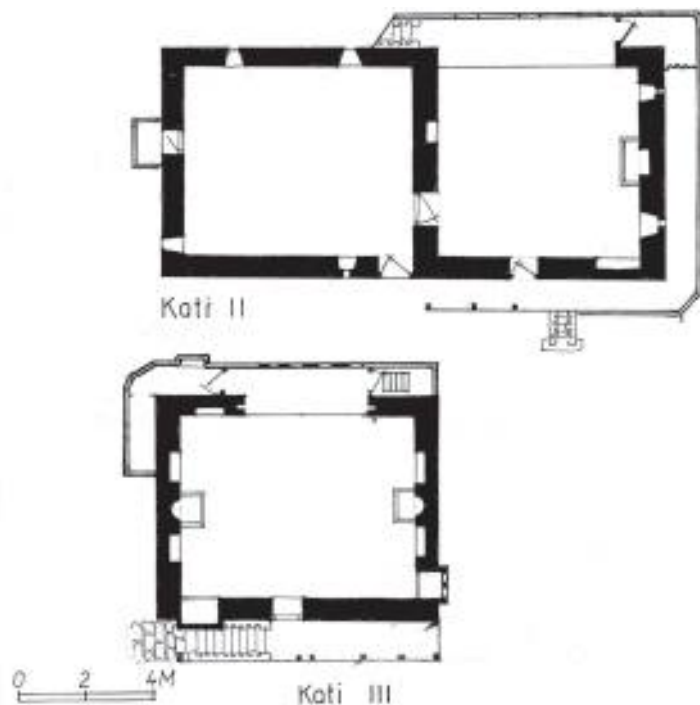
Fig. 443-445. Zdrajsh, Çermenikë-Librazhd. Rritja numerike dhe fuqizimi ekonomik i familjes kanë krijuar mundësinë e ngritjes së një ndërtimi të ri trikatësh, ngjitur me banesën e vjetër dykatëshe. Në katin e tretë të ndërtimit të ri ka kaluar oda e miqve.
