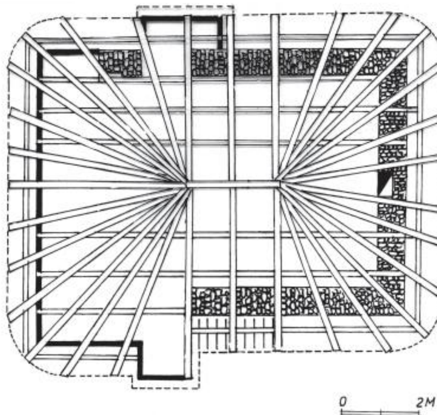
Fig. 175. Has-Kukës. Detaje konstruktive. Kapja e trarëve me njëri-tjetrin bëhet me kllapa, duke e bërë njëjën rigjide, pa pasur nevojë për përdorimin e gozhdëve.
