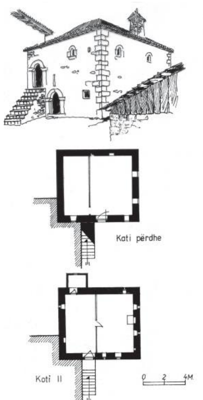
Fig. 222-223. Bozhë, Lumë-Kukës. Varianti më i thjeshtë i tipit të mbyllur. Banesa është dykatëshe, me nga një kthinë në çdo kat. Hyrjet për çdo mjedis janë të veçanta ku ajo e katit përdhes mbrohet nga një frëngji e hapur sipër saj.
