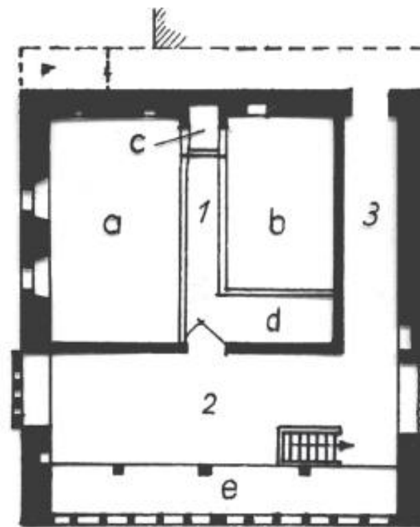
Fig. 160. Skema kompozicionale e katit të sipërm të banesës dhe e dhomës së miqve është e tipizuar për të gjitha variantet e banesës, qofshin ato përdhese, me dy ose tre kate.
