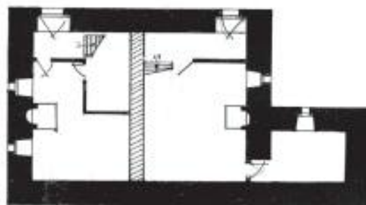
Koti përdhe
