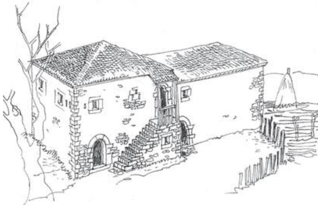
Fig. 85. Kallmet, Zadrimë-Lezhë. Banesës njëkthinëshe dykatëshe i është bashkangjitur, në një kohë më të vonë, një bërthamë dykatëshe. Të dy njësitë lidhen së brendëshmi me njëra-tjetrën. Njësia e parë është më e përpunuar nga ana arkitektonike. Kthina e katit është pajisur me shumë frëngji për mbrojtje.
