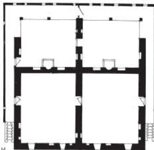
Kati III
