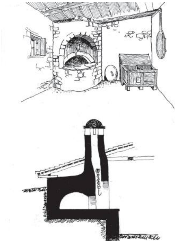
Fig. 49. Kryezi-Pukë. Furrë buke në shtëpinë e zjarrit. Në këtë rast ajo është e pajisur me kanal tymi. Përdorej për pjekje dhe gatim. Përpara portës së furrës është zgjatur praku ku tërhiqej një pjesë e zjarrit. Aty ngrohet ushqimi e mbi të varen enët për gatim.
