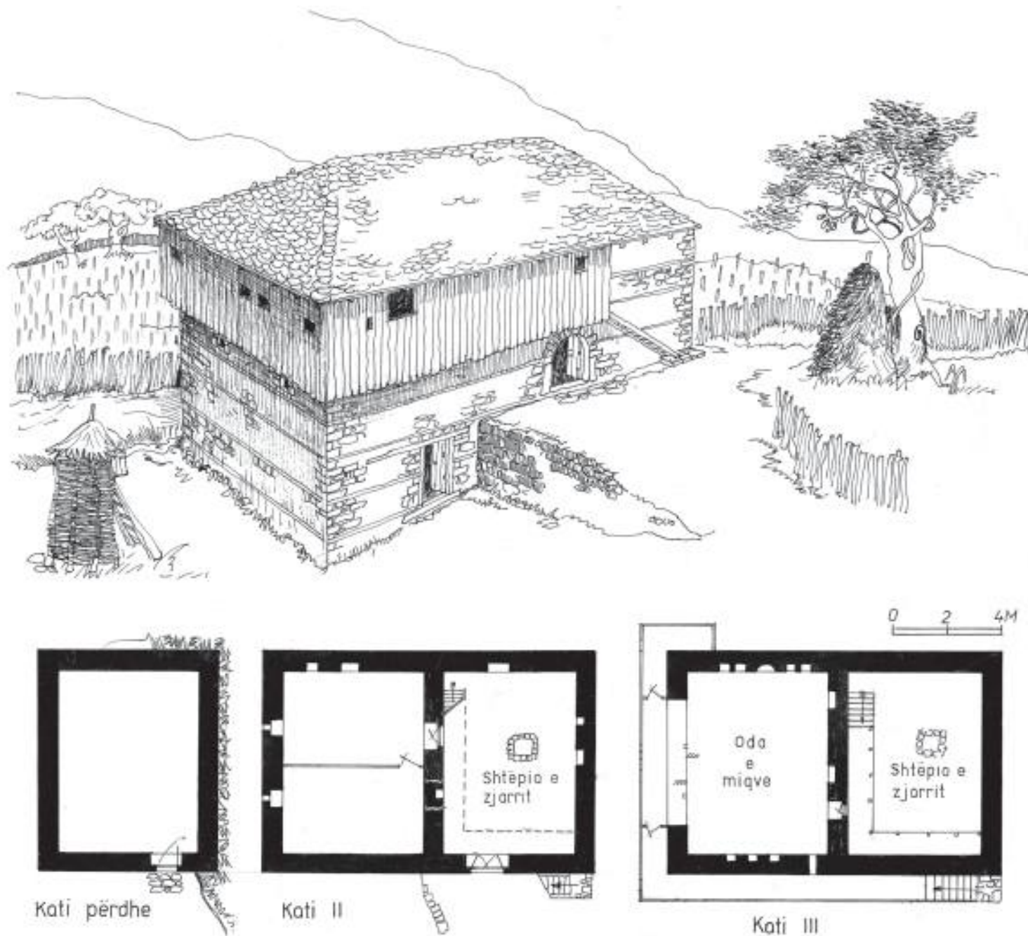
Fig. 430. Bastar i Mesëm, Malësia e Tiranës-Tiranë. Zhvillimi i banesës ka rrjedhur si rezultat i shtrirjes së saj tërthor rënies së terrenit. Pjesa balllore trikatëshe ka ruajtur kompozimin njëkthinësh, ndërsa në pjesën e prapme është vendosur shtëpia e zjarrit.
