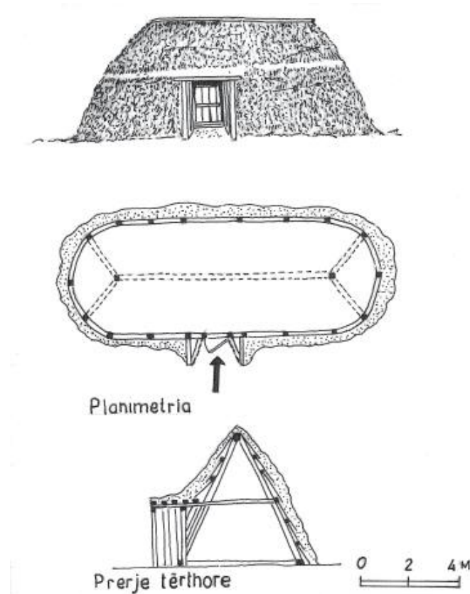
Fig. 31. Arst, Brigjet-Pukë. Pojatë. Është ndërtuar me skelet druri, i mbuluar me degë për kullimin e ujrave. Shtresa e dheut shërben si termoizoluese dhe mbrojtëse e mjedisit nga erërat e këqija (pamje, planimetri, prerje).
