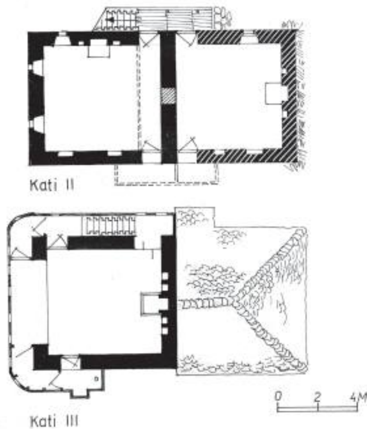
Fig. 423-424. Dranovicë (Kostenjë), Çermenikë-Librazhd. Në ndërtimin përdhës të shtuar më vonë ka kaluar shtëpia e zjarrit.
