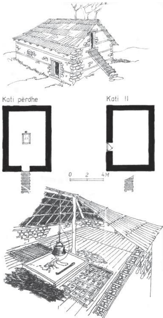
Fig. 279-280. Peshk, Martanesh- Mat. Kasollja e stanit është e ndërtuar me gurë, kati përdhes i të cilës përdorej për strehimin e kafshëve të ngarkesës dhe hapsira nën çati për banimin e barinjve.
