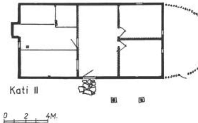
Fig. 133-134. Vranisht, Has-Kukës. Shtëpia e zjarrit, është ndërtimi i parë nga zuri fill zhvillimi i mëtejshëm i kompleksit. Përmasat e mëdha dhe kompozimi në gjysmëkat kanë lejuar që aty të përfshihen të gjitha mjediset e nevojshme për plotësimin e nevojave të familjes: gatimi, pritja, fjetja dhe strehimi i bagëtive. Vëllimi i poshtëm, është i futur në tokë.
