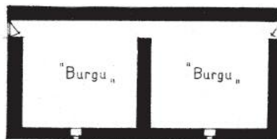
Kati përdhe
