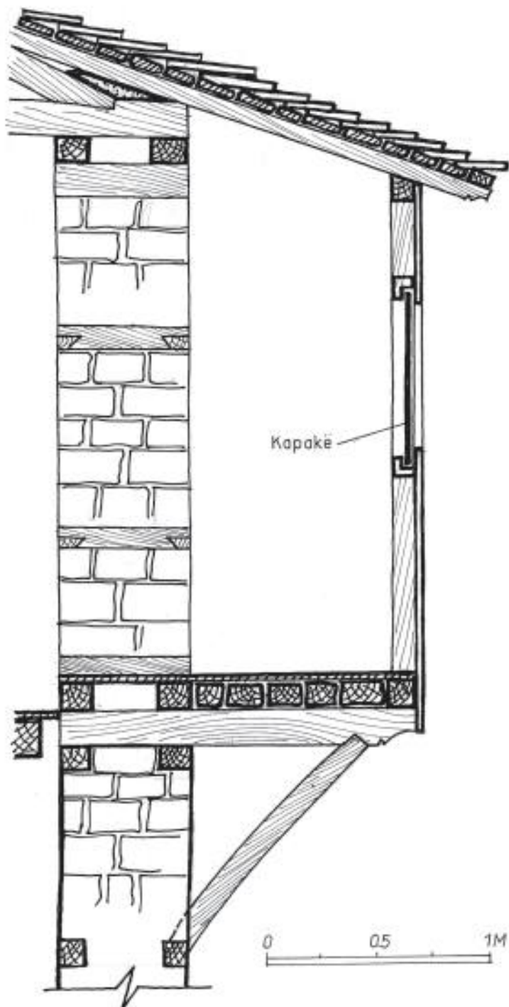
Fig. 489-490. Në disa zona fshatare ku kanë gjetur përdorim qoshqet, mjeshtri i ka kushtuar vëmendje konstruksionit mbajtës të tyre.
