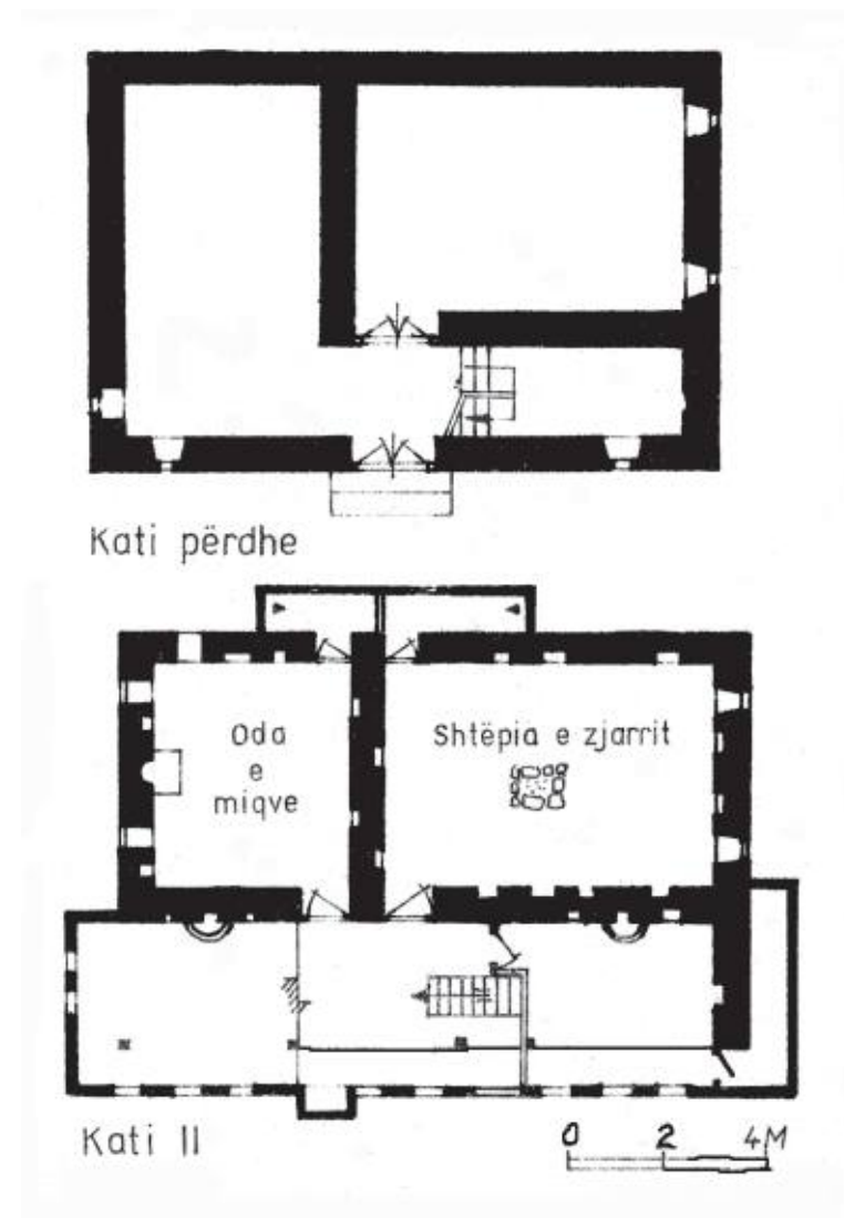
Fig. 358-359. Herbel-Dibër. Banesë dykatëshe me zhvillim gjatësor, me tri mjedise radhazi, të paraprirë nga një treme e hapur në faqen gjatësore të katit. Në një kohë të mëvonshme krahu i majtë i shtëpisë ka pësuar ndryshime, si pasojë e ndarjes së familjes. Në pjesën e paprekur nga ndryshimet, çardaku ka sipërfaqe të madhe, është i mbrojtur në të dy anët e ngushta nga zgjatimi i mureve anësorë të banesës dhe përdorej edhe si vend pune. Ngjitur me parapetin e ballit të hapur janë ndërtuar koshi i drithit dhe hambaret.
