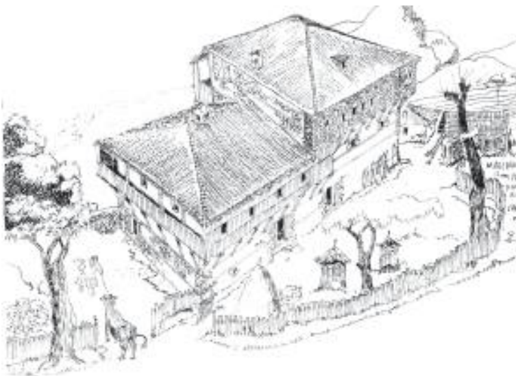
Fig. 443-445. Zdrajsh, Çermenikë-Librazhd. Rritja numerike dhe fuqizimi ekonomik i familjes kanë krijuar mundësinë e ngritjes së një ndërtimi të ri trikatësh, ngjitur me banesën e vjetër dykatëshe. Në katin e tretë të ndërtimit të ri ka kaluar oda e miqve.
