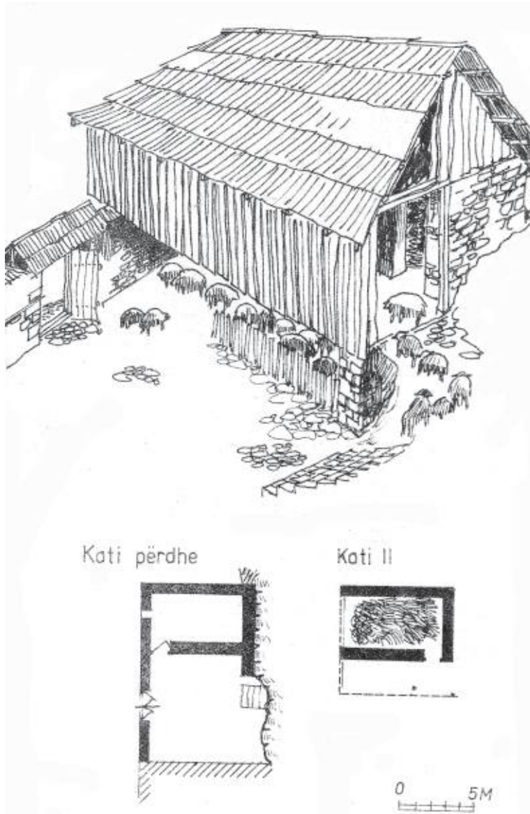
Fig. 295. Lenë, Martanesh-Mat. Kasolle bari e gjaje. Është vendosur në terren të pjerrët. Në katin përdhe, gjysmë të futur në tokë, mbaheshin bagëtitë dhe në hajatin përpara tij drutë e zjarrit. Në nivelin e sipërm, galeria e veshur me dërrasa përdorej për strehimin e kecape, ndërsa e ndara tjetër dhe hapësira nën çati për depozitimin e barit.
