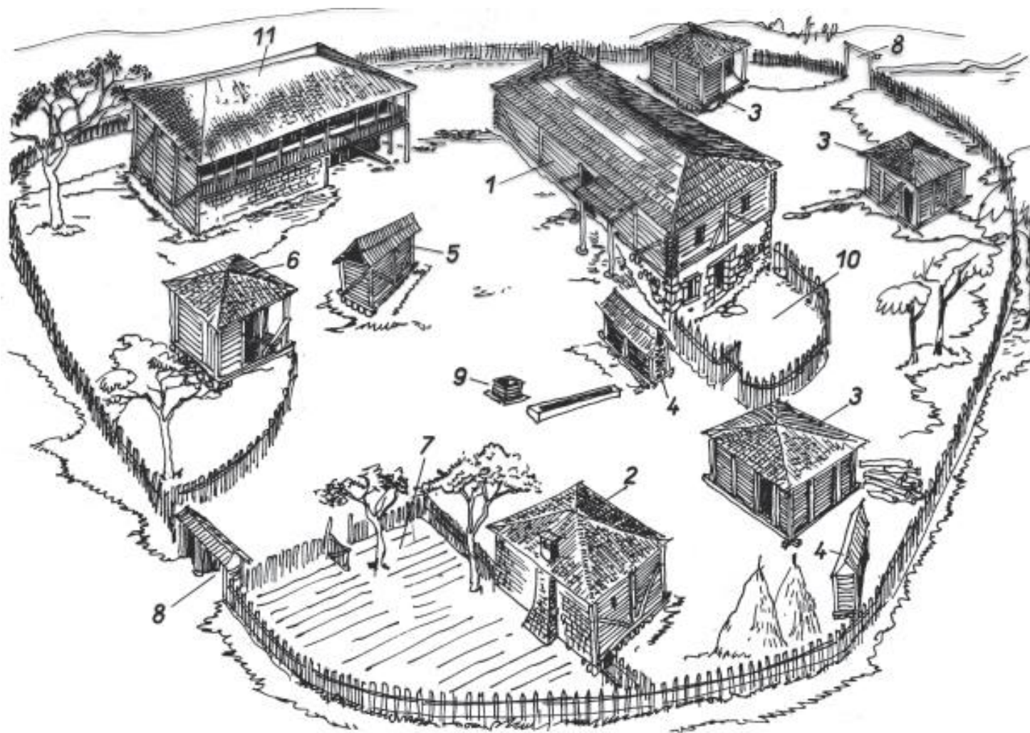
Fig. 132. Vranisht, Has-Kukës. Grupimi i ndërtimeve të një familjeje të madhe; 1. Shtëpia e zjarrit; 2. Shtëpia e mique; 3. Qilerët; 4. Koshar misri; 5. Çaraniku i bulmetit; 6. Hambari; 7. Kopështi i perimeve; 8. Portat e oborrit; 9. Pusi me koritën; 10. Vathë për bagëtinë; 11. Ndërtimi i ri i familjes. Ndërtimi kryesor që formon qendrën kompozicionale të kompleksit, është shtëpia e zjarrit, ndërtimet e tjera banimi ose ekonomike, e rrethojnë atë.
