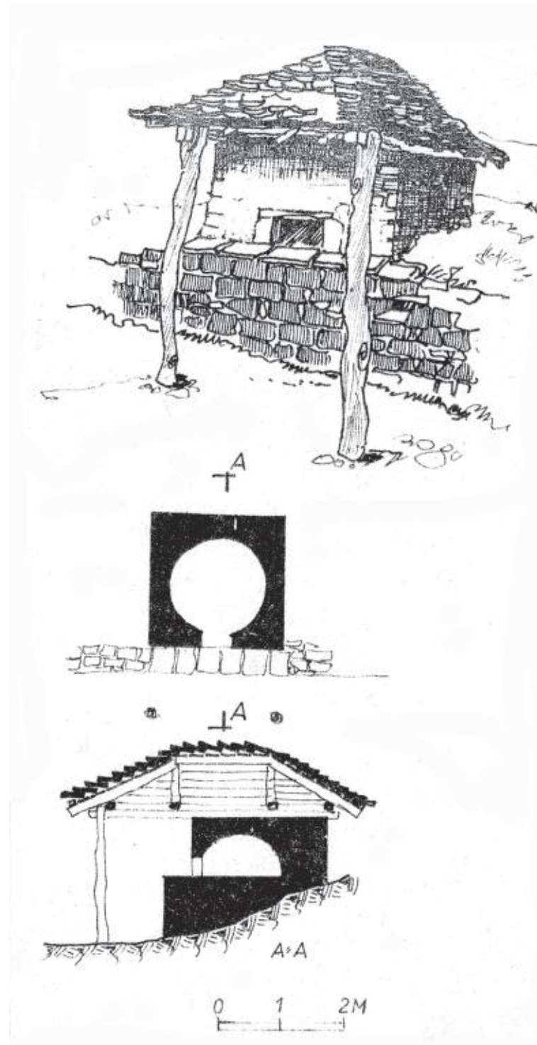
Fig. 309. Çermenikë-Librazhd. Shtreth për depozitimin e barit. Mullari ngrihet mbi një konstruksion druri, duke krijuar poshtë tij një hapsirë të mbrojtur.
