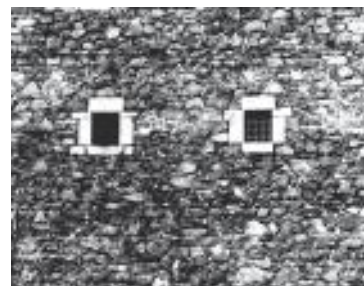
Fig. 474-475 a, b. c. Teknika e muraturës me gurë të lidhur me llaç gëlqere, pavarësisht zonës ku zbatohej realizohej pa breza druri ose i kishte ata të “fshehur” në trashësinë e murit.
