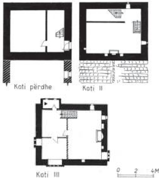
Fig. 419-420. Kurbnesh-Mirditë. Kërkesat që lindin nga rritja e familjes shpesh nuk mund të përballohen nga mjediset ekzistuese edhe në banesat trikatëshe. Në hapësirën e tyre veçohen kthina të vogla (si ajo në katin e tretë), ose vëllimit fillestar i shtohet një ndërtim i ri, zakonisht përdhes, ku kalon shtëpia e zjarrit.
