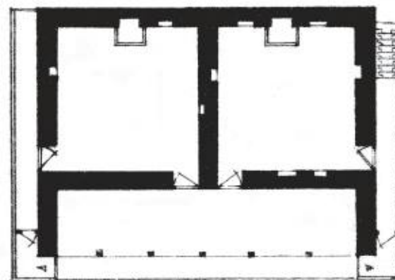
Kati II
