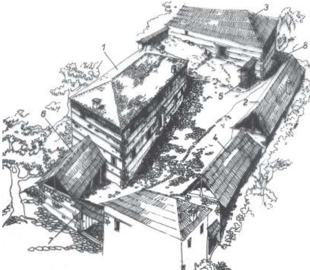
Fig. 289-290. Radomirë-Dibër. 1. Banesa; 2. Vatra dhe quri i bulmetit; 3, 4. Pojata; 5. Gazhdari; 6. depoja e druve; 7. Porta kryesore; 8. Porta e kopshtit. Ndërtimet ndihmëse janë mbledhur rrotull banesës, pothuajse ngjitur me njeri-tjetrin duke krijuar oborrin, që kryesisht ka funksione ndërlidhëse. Ky i fundit është i shtruar me kalldrëm. Banesa zë vendin qendror në kompozimin e asambliit.
