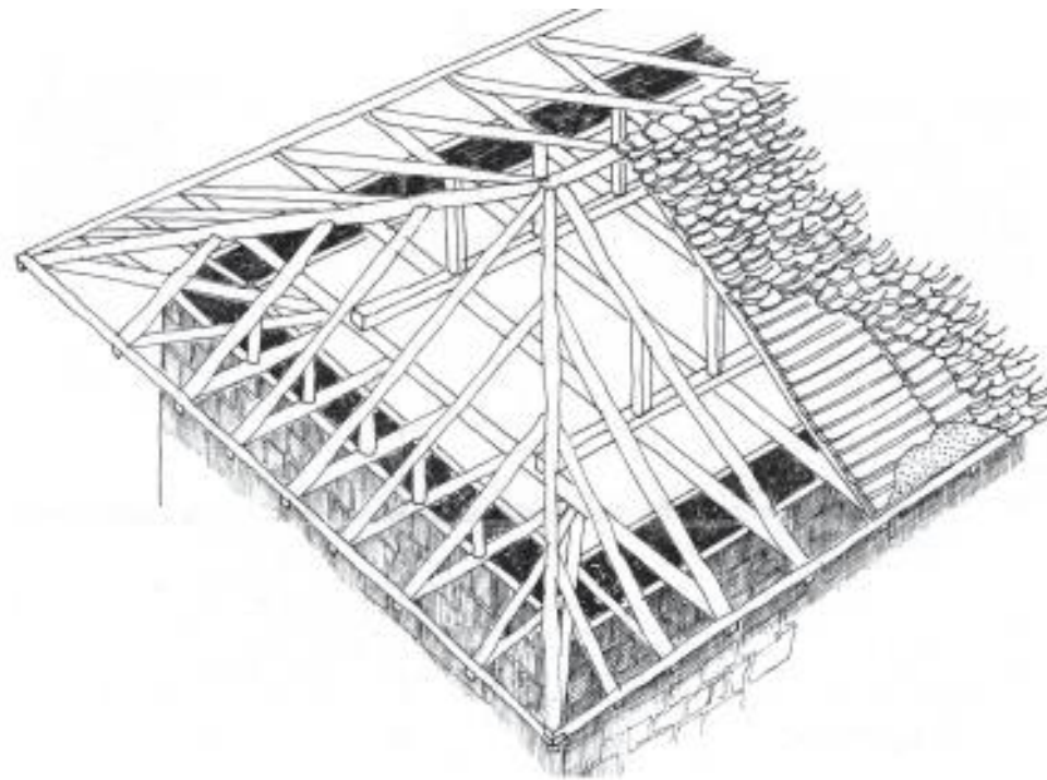
Fig. 480. Konstruktion çatie me lëndë të rrumbullakët. Është zbatuar në mjaft zona të vendit. Diametri i elementeve ndryshonte në varësi të rolit dhe të vendit që zinin në konstruktionin mbajtës të çatisë.
