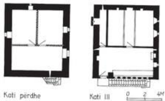
Fig. 197-198. Helshan, Has-Kukës. Banesë dykatëshe e ndërtuar tërësisht me gurë.
