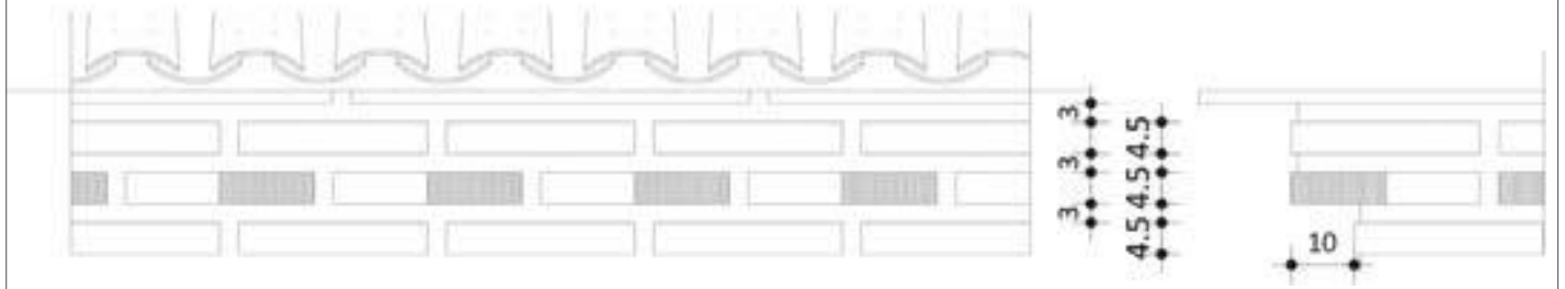
Fig. 29. Detaj i kornizës me një radhë në formë dhëmbësh sharre
