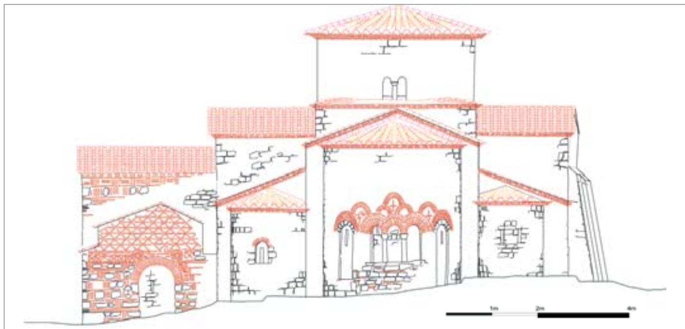
Fig. 38. Propozimi për pamjen lindore të kishës
