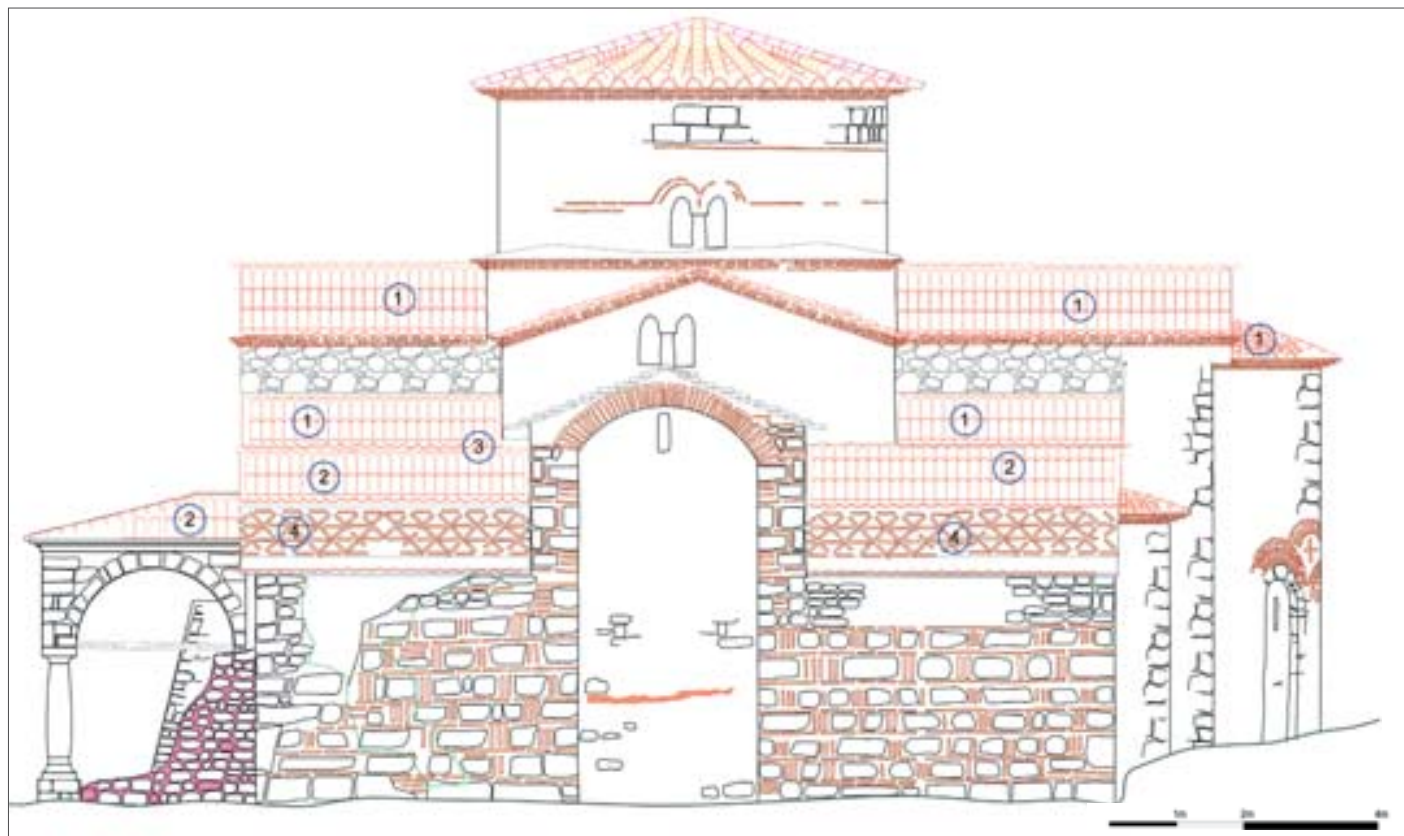
Fig. 39. Propozimi për pamjen jugore të kishës
