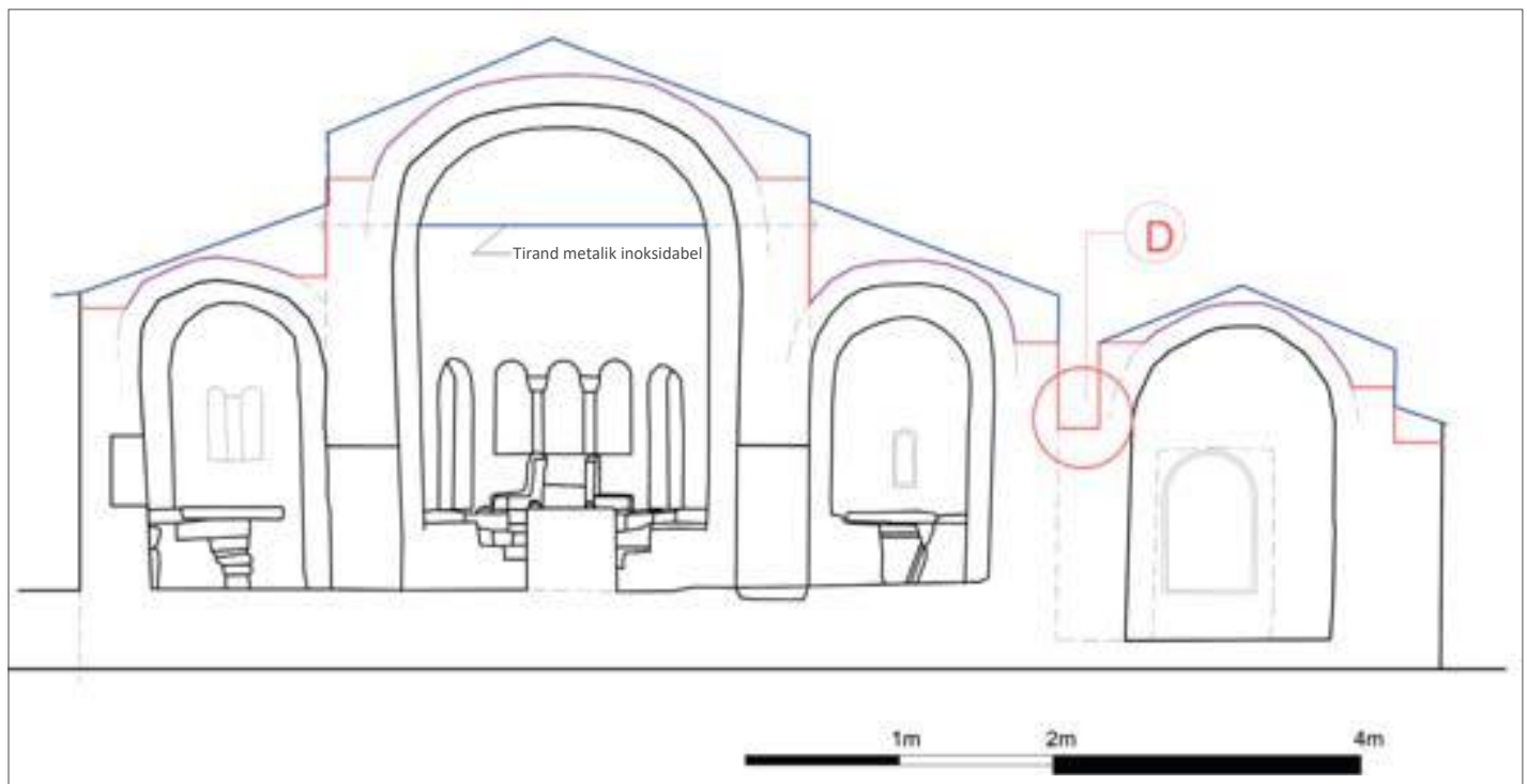
Fig. 28. Konfiguracioni i mbulesës fillestare të anës lindore
