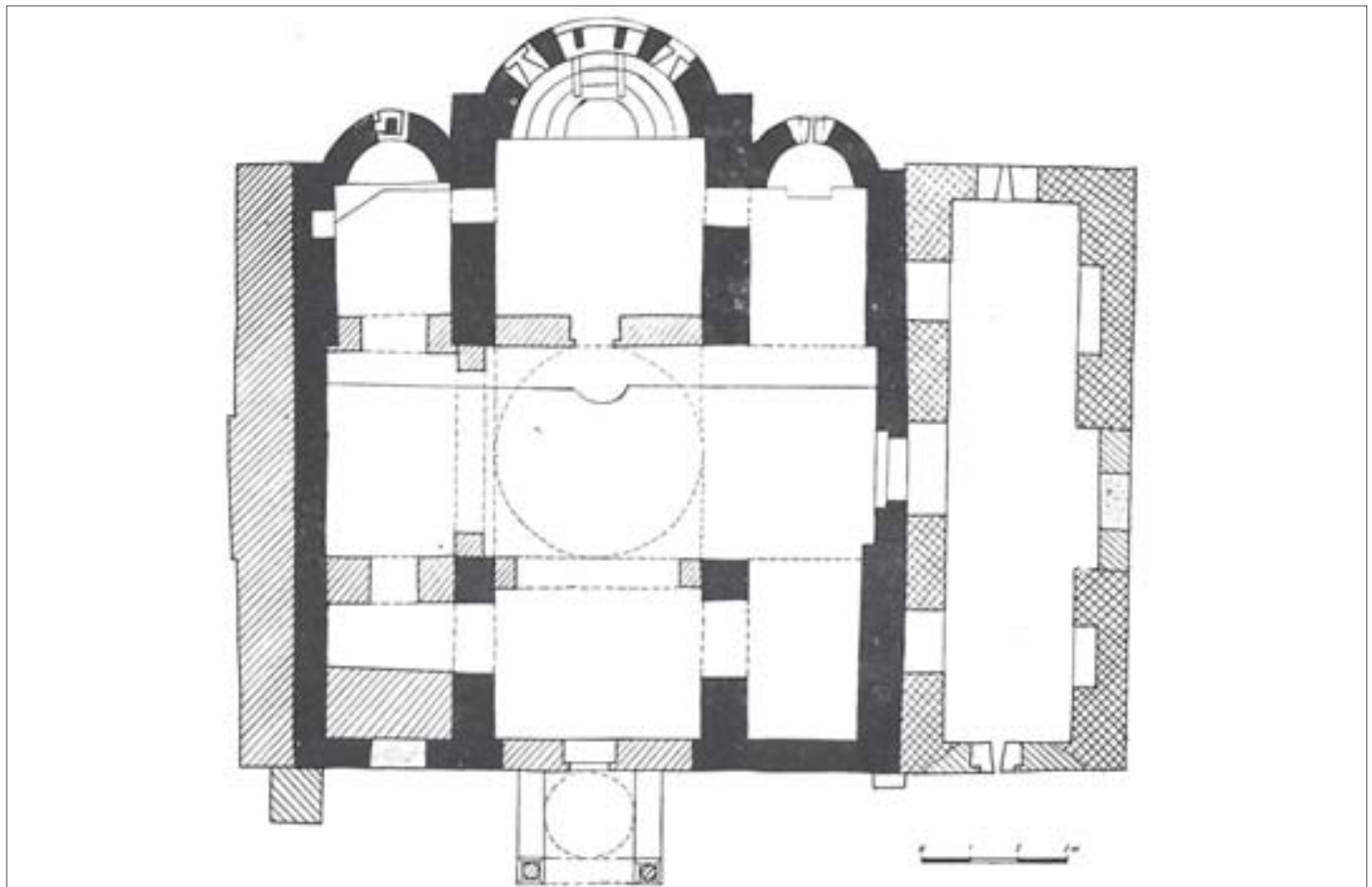
Fig. 3. Planimetria
