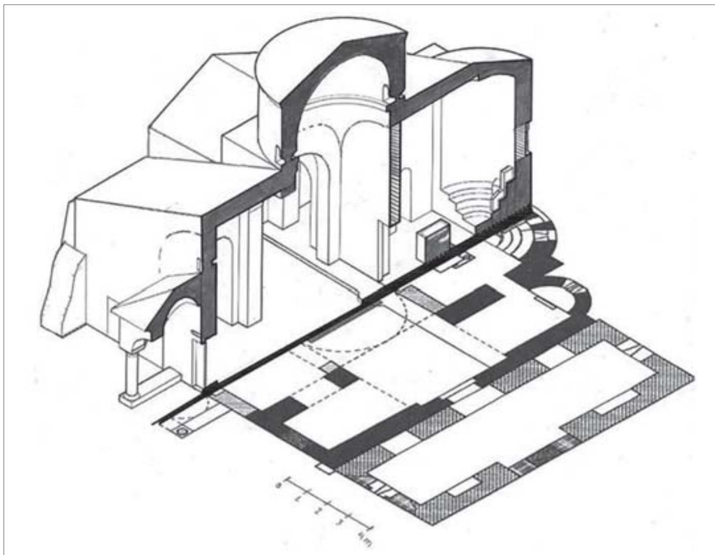
Fig. 4. Prerja aksonometrike
