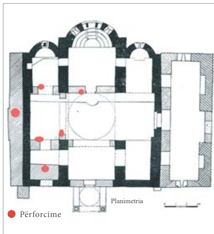
Fig. 12. Përforcimet e kryera në kohë
