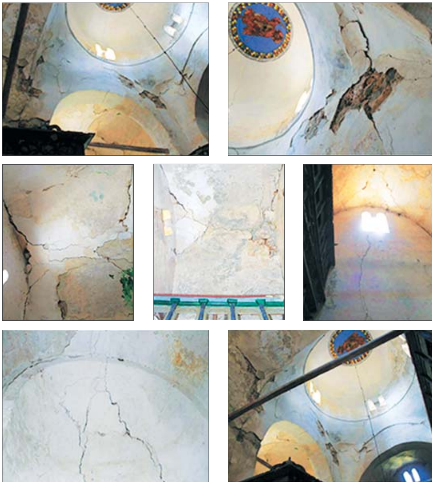
Fig. 42. Dëmtimet e strukturës së kurbëzuar të mbulesës
