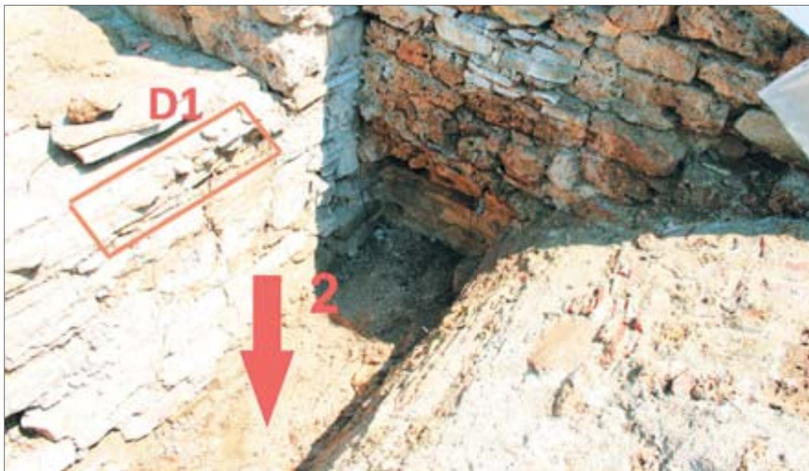
Fig. 20. Zbulimi i ullukut ndërmjet mbulesës së fazës së parë dhe shtesës jugore në anën perëndimore
