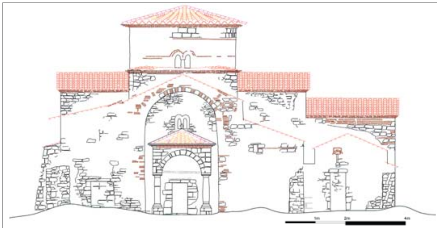
Fig. 37. Propozimi për pamjen perëndimore të kishës
