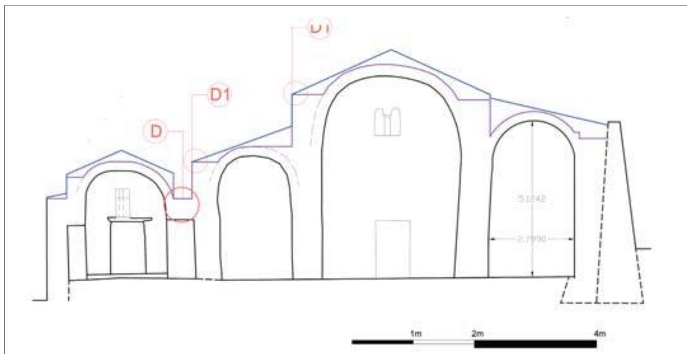
Fig. 23. Konfiguracioni i mbulesës fillestare të anës perëndimore
