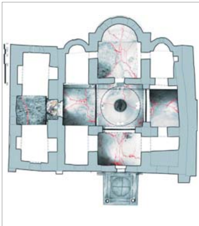
Fig. 14. Dëmtimet e sistemit të mbulesës
